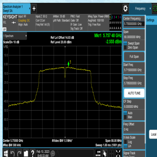
11N40SISO-Ant1-5755--5.04-0.26-2.22-0.00
