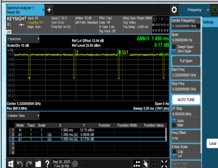
NTNV-11A-Ant0-5320
