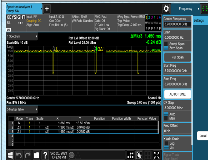
NTNV-11A-Ant0-5700
