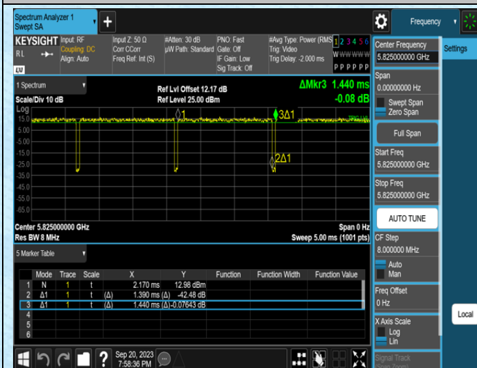
NTNV-11A-Ant0-5825
