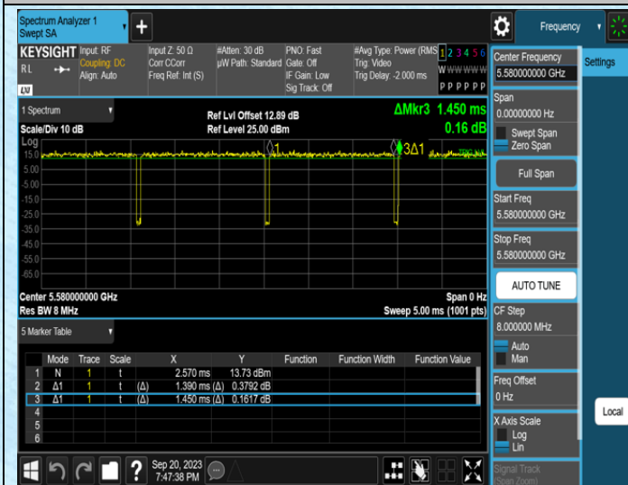
NTNV-11A-Ant0-5580
