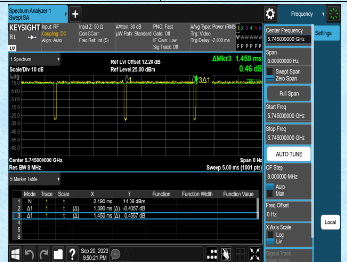
NTNV-11A-Ant1-5745
