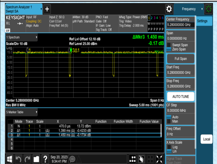
NTNV-11A-Ant1-5280
