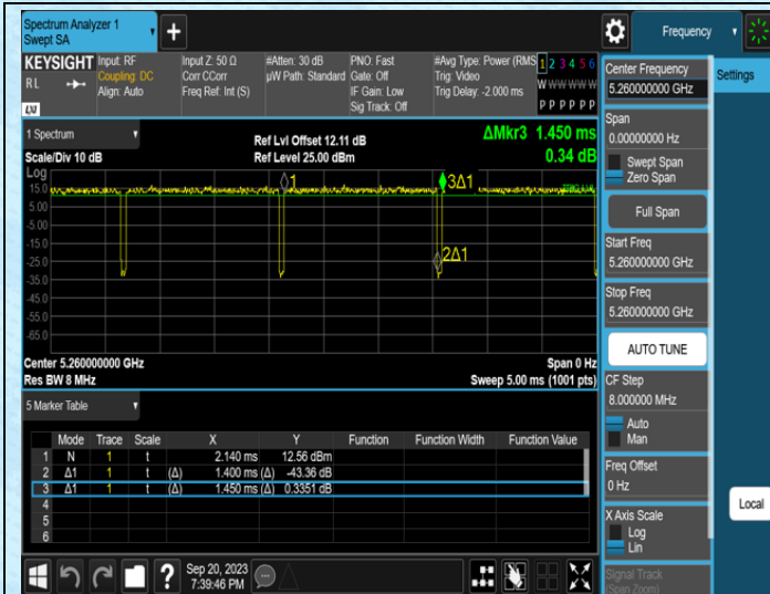
NTNV-11A-Ant0-5260
