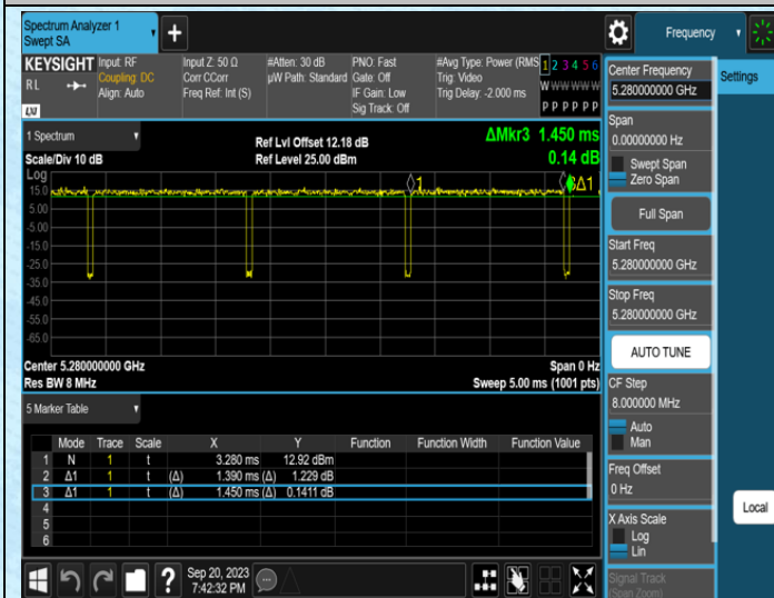
NTNV-11A-Ant0-5280
