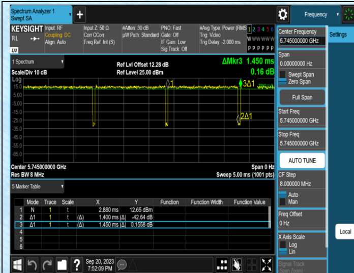
NTNV-11A-Ant0-5745
