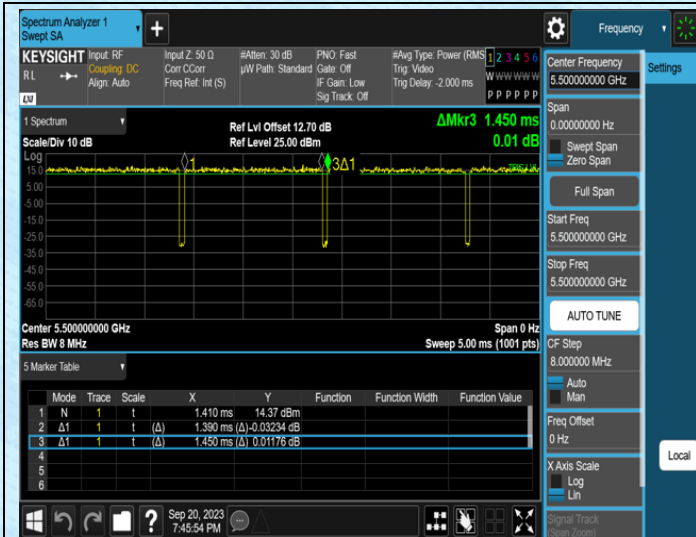
NTNV-11A-Ant0-5500
