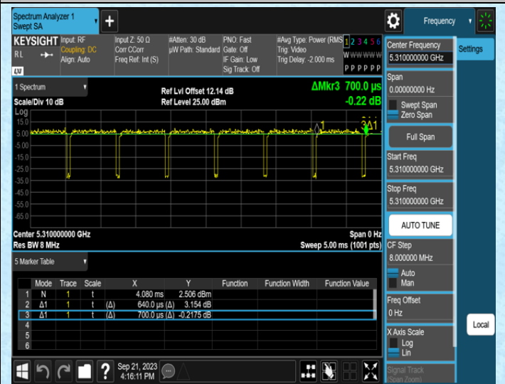
NTNV-11N40MIMO-Ant1-5310
