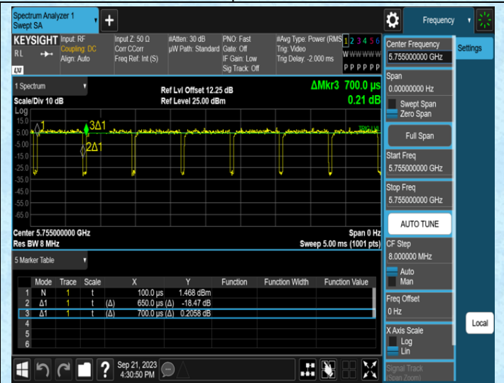
NTNV-11N40MIMO-Ant1-5755
