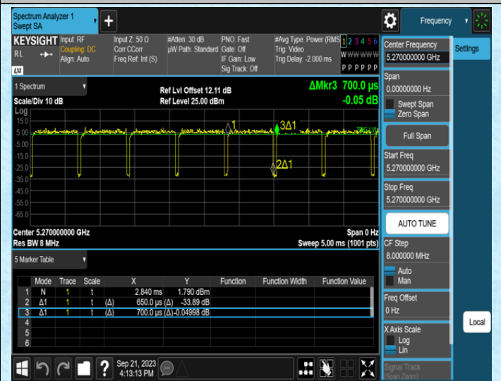
NTNV-11N40MIMO-Ant1-5270
