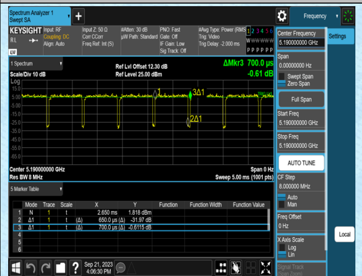
NTNV-11N40MIMO-Ant1-5190
