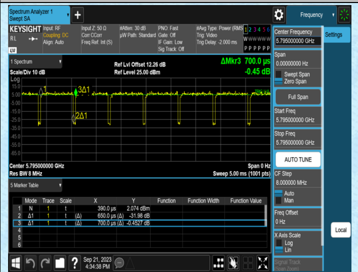
NTNV-11N40MIMO-Ant1-5795
