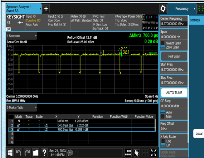
NTNV-11N40MIMO-Ant0-5270
