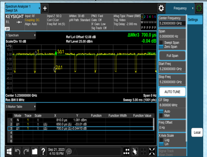
NTNV-11N40MIMO-Ant1-5230
