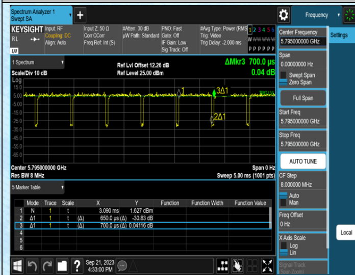
NTNV-11N40MIMO-Ant0-5795
