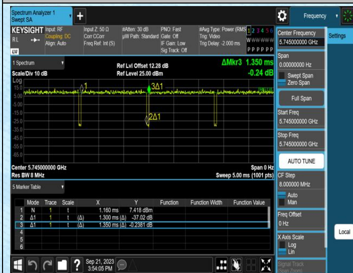
NTNV-11N20MIMO-Ant0-5745
