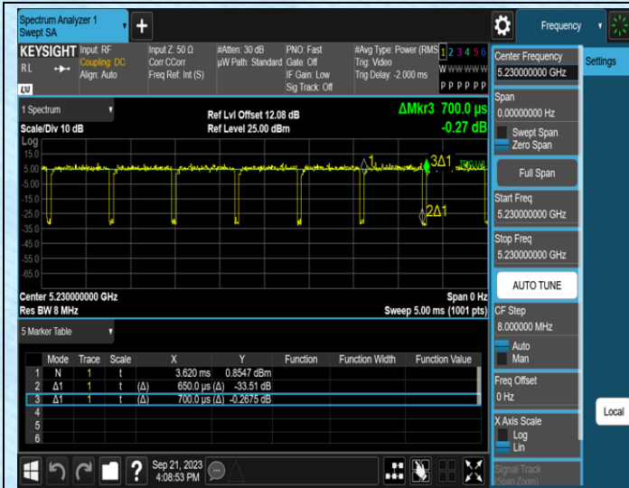
NTNV-11N40MIMO-Ant0-5230
