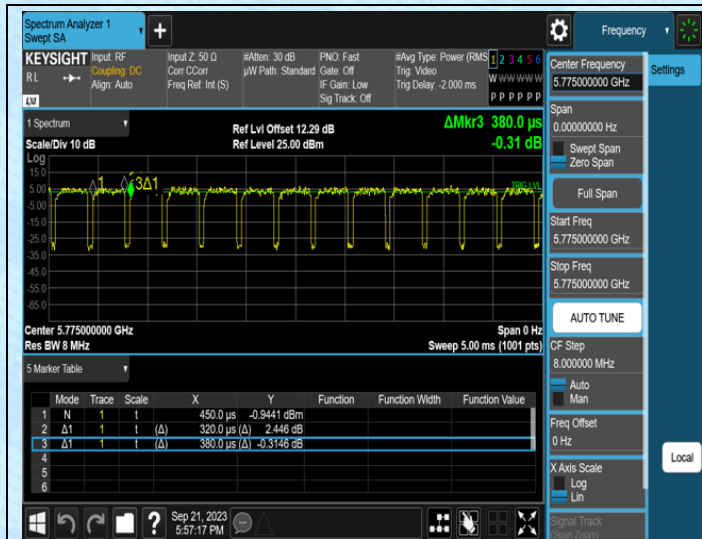
NTNV-11AC80MIMO-Ant0-5775
