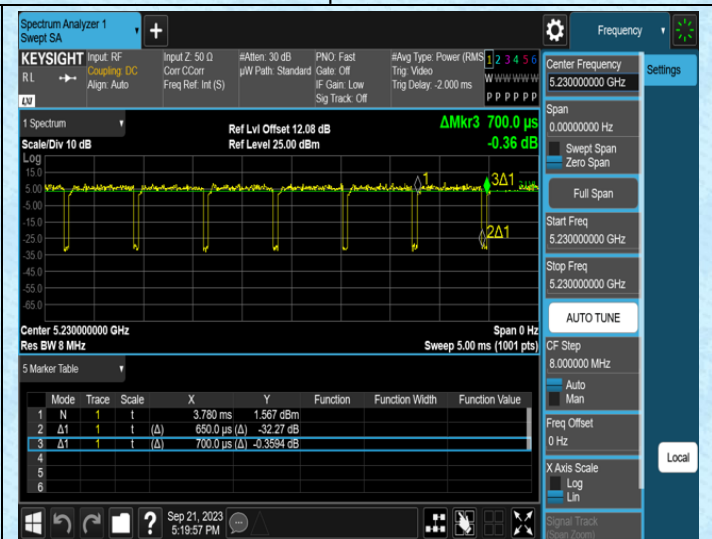
NTNV-11AC40MIMO-Ant1-5230
