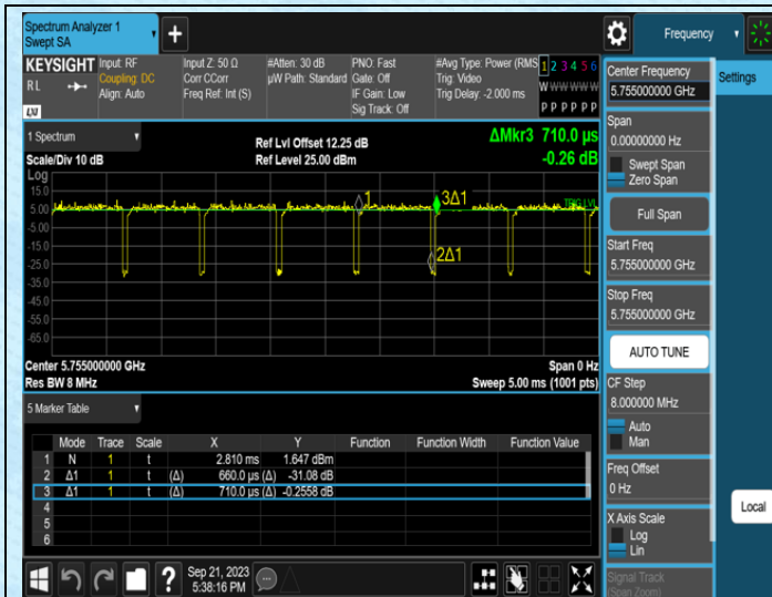
NTNV-11AC40MIMO-Ant0-5755
