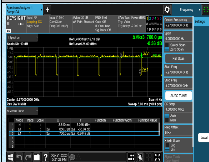
NTNV-11AC40MIMO-Ant0-5270
