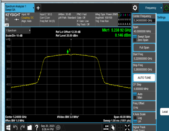
11N20SISO-Ant0-5240
