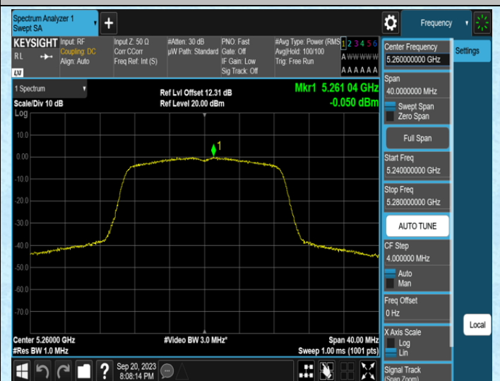
11N20SISO-Ant0-5260
