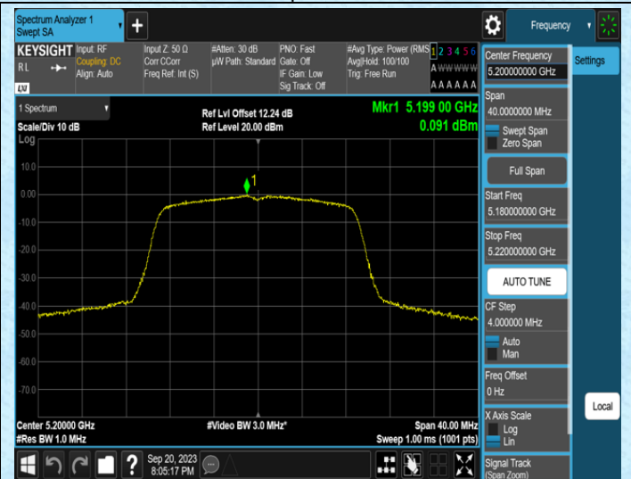
11N20SISO-Ant0-5200
