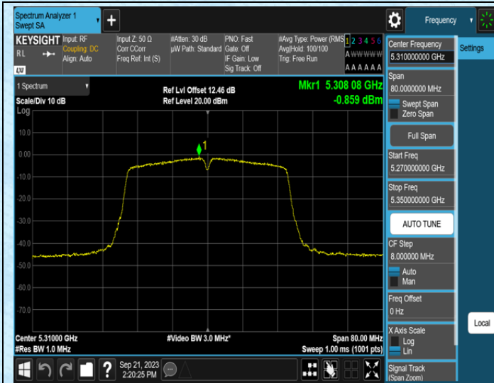
11N40SISO-Ant1-5310
