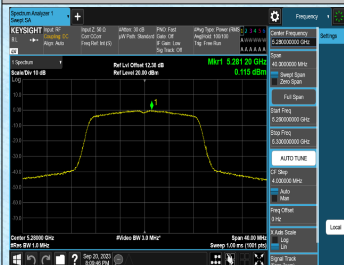
11N20SISO-Ant0-5280
