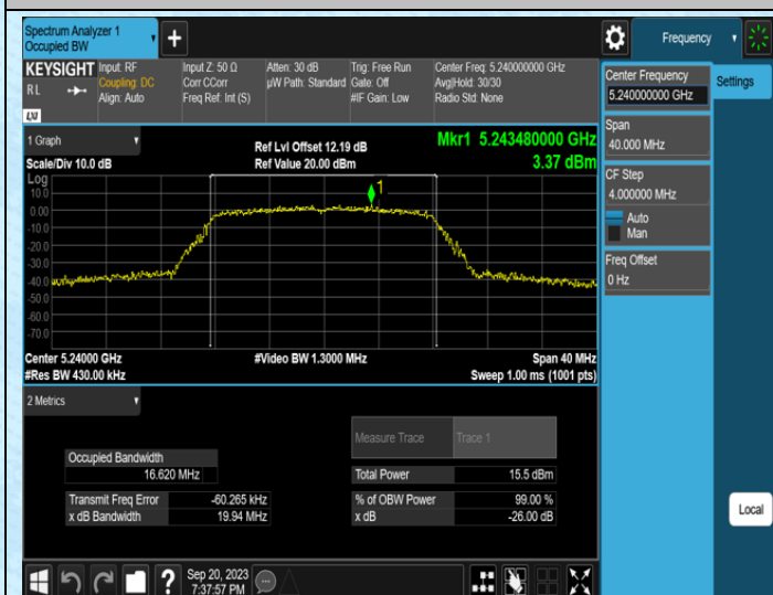
11A-Ant0-5240
