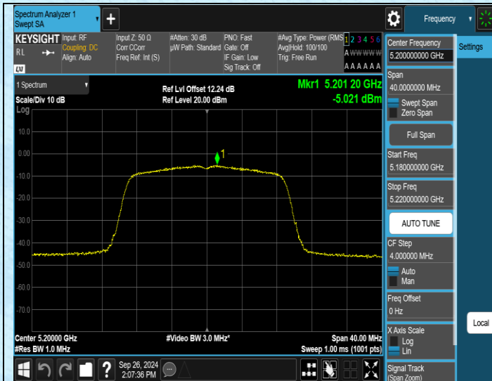
11N20MIMO-Ant1-5200-PASS
