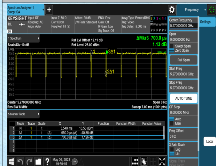
NTNV-11N40MIMO-Ant1-5270
