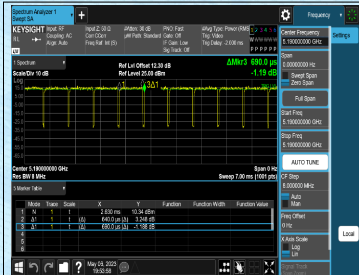
NTNV-11N40MIMO-Ant1-5190
