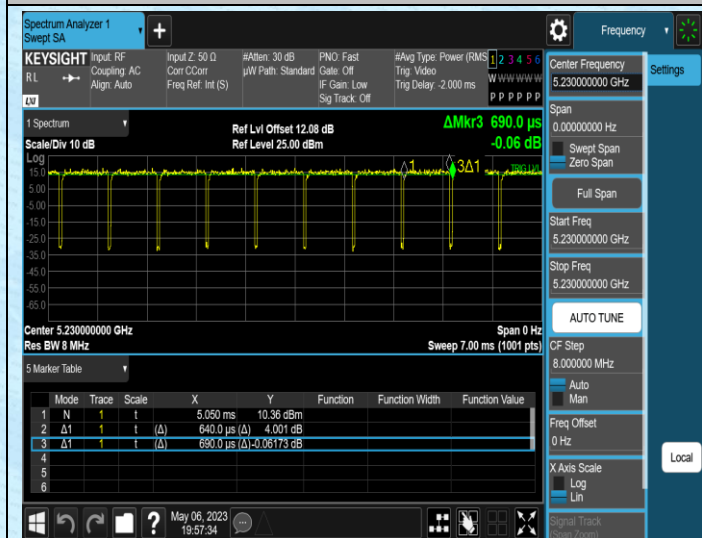
NTNV-11N40MIMO-Ant1-5230
