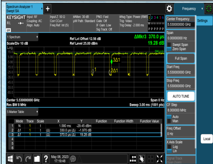
NTNV-11AC80SISO-Ant1-5530
