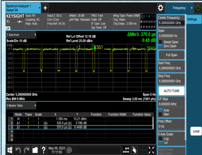
NTNV-11AC80SISO-Ant1-5290
