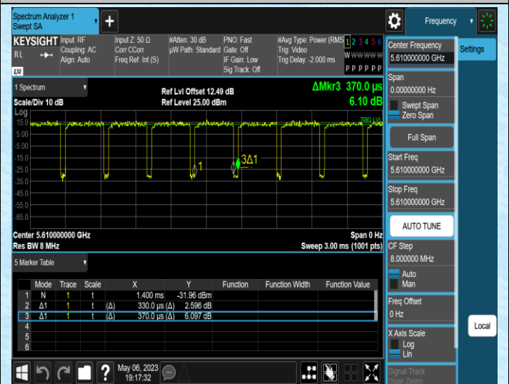
NTNV-11AC80SISO-Ant2-5610
