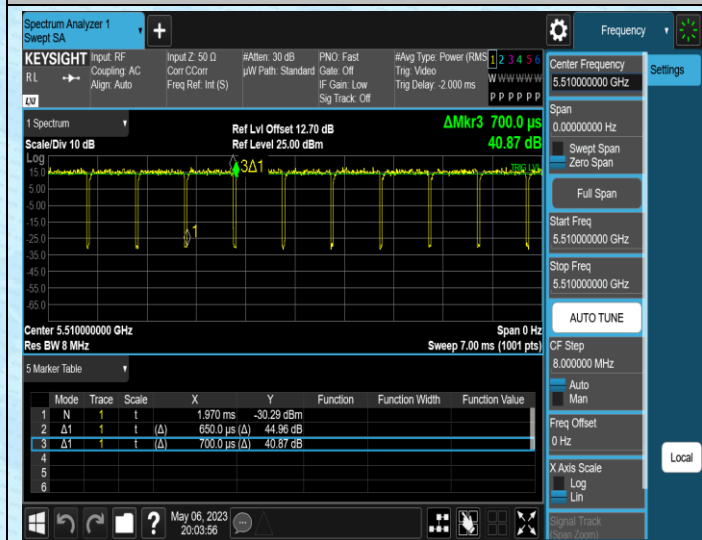
NTNV-11N40MIMO-Ant1-5510
