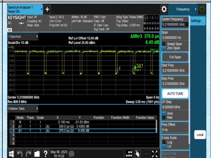
NTNV-11AC80SISO-Ant2-5210
