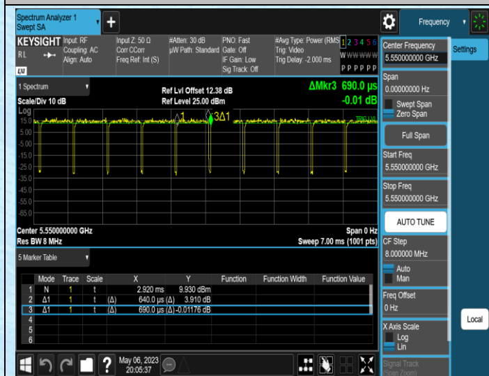
NTNV-11N40MIMO-Ant1-5550
