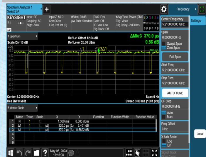
NTNV-11AC80SISO-Ant1-5210
