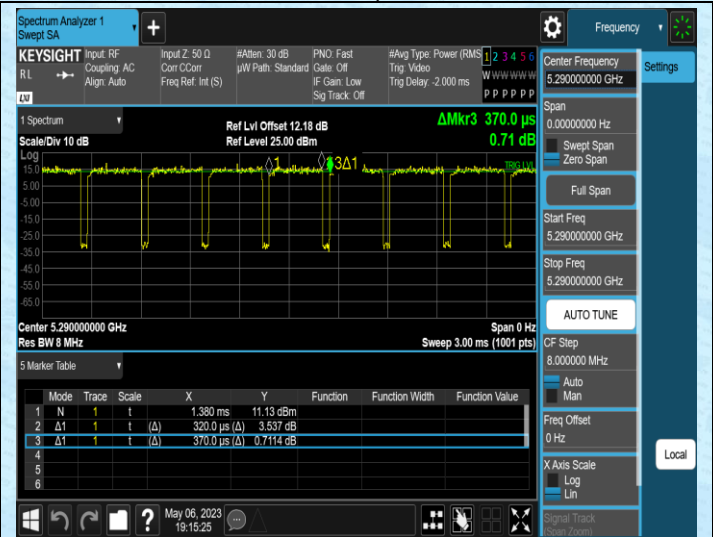
NTNV-11AC80SISO-Ant2-5290
