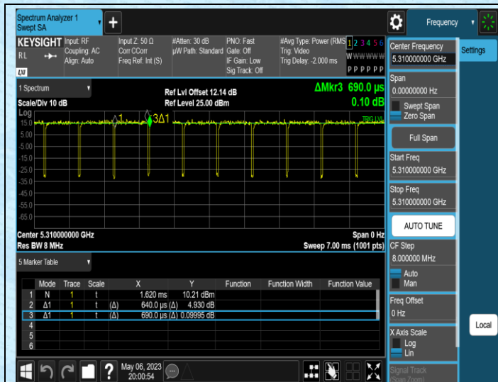
NTNV-11N40MIMO-Ant1-5310
