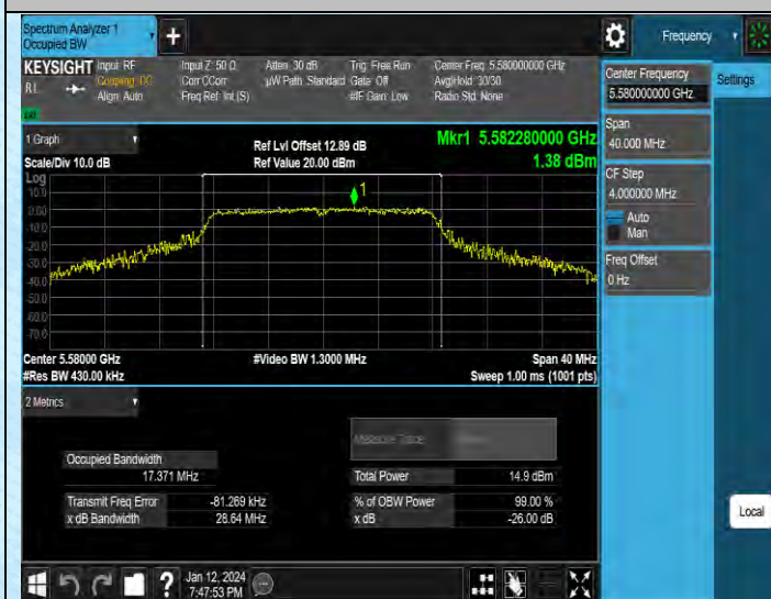
11A-Ant1-5580
