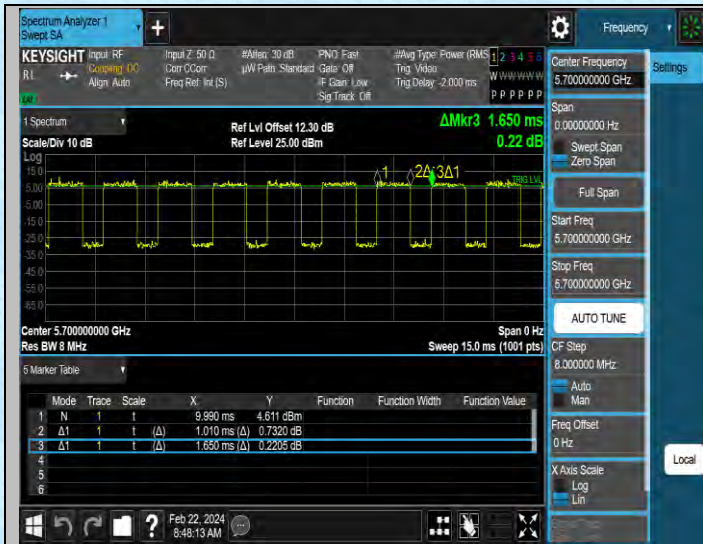
NTNV-11AX20MIMO-Ant1-5700
