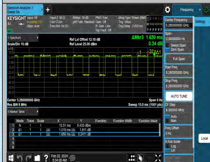
NTNV-11AX20MIMO-Ant1-5280
