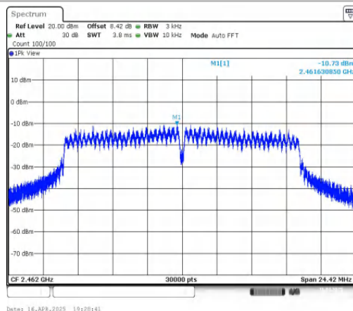
11G-CDD-Ant2-2462-PASS
