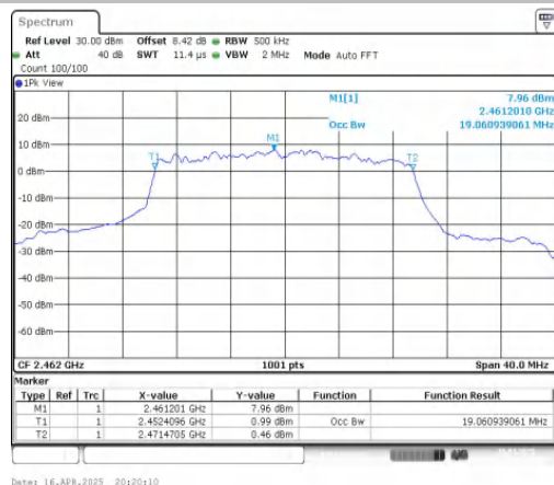
11AX20MIMO-Ant2-2462
