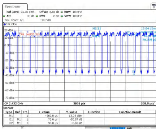
NTNV-11AX40MIMO-Ant1-2422
