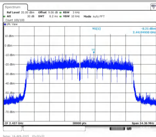
11AX40MIMO-Ant1-2437-PASS
