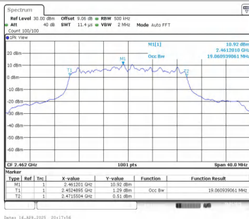
11AX20MIMO-Ant1-2462
