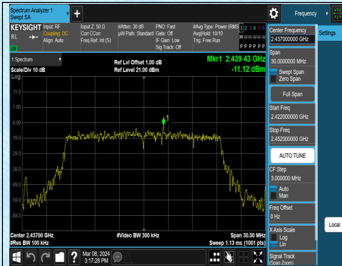
11AX20MIMO-Ant1-2437-0-Reference-PASS
