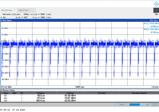
802.11ax HE80_5210MHz
