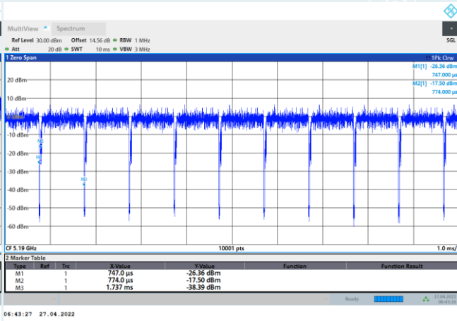
802.11ax HE40_5190MHz
