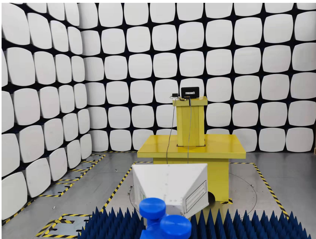
RSE (1-18) GHz
