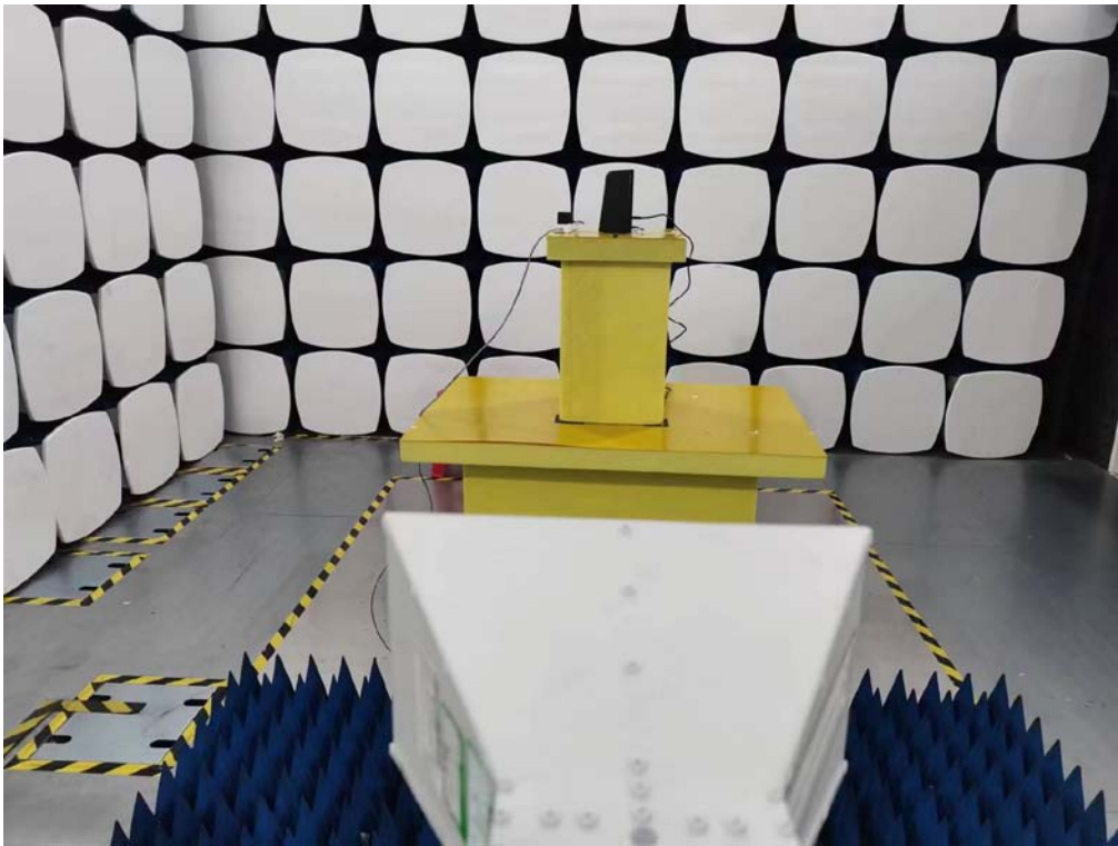
RSE (1-18) GHz
