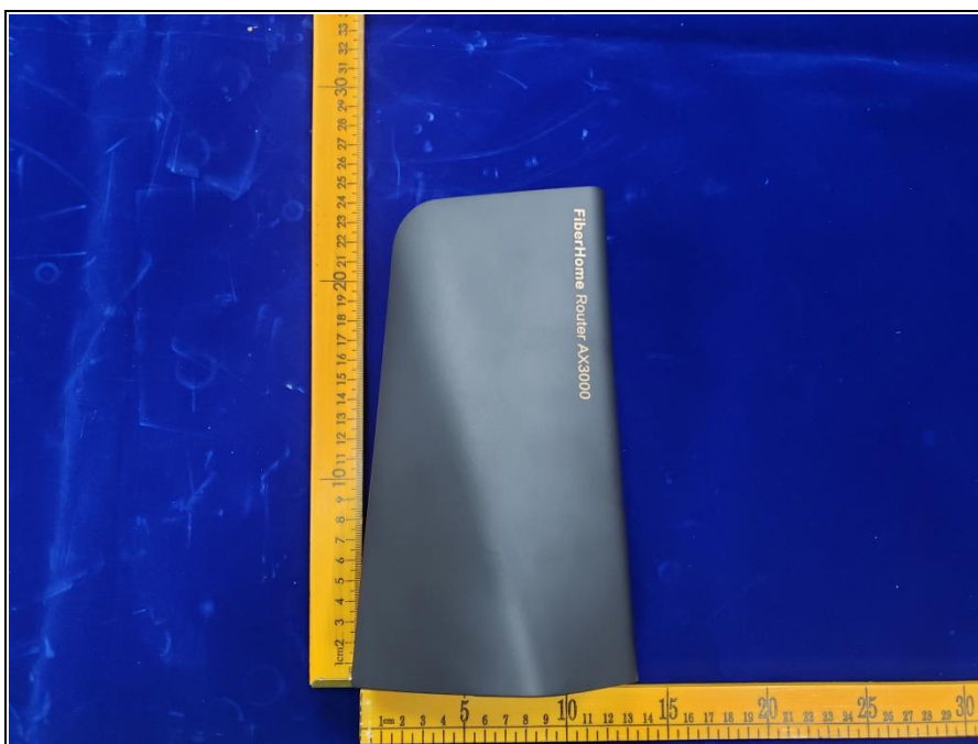
EUT-2
