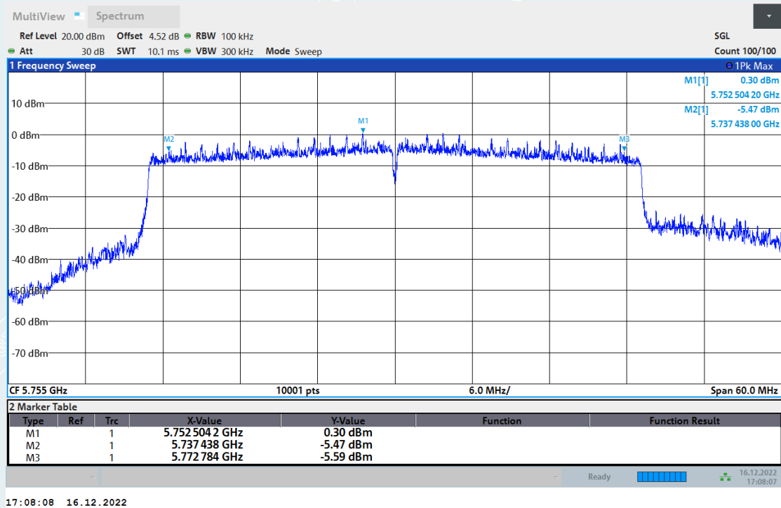
6dB Bandwidth NVNT ax40 5755MHz Ant1
