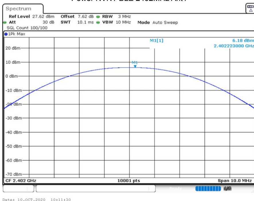
Power NVNT BLE 2402MHz Ant1
