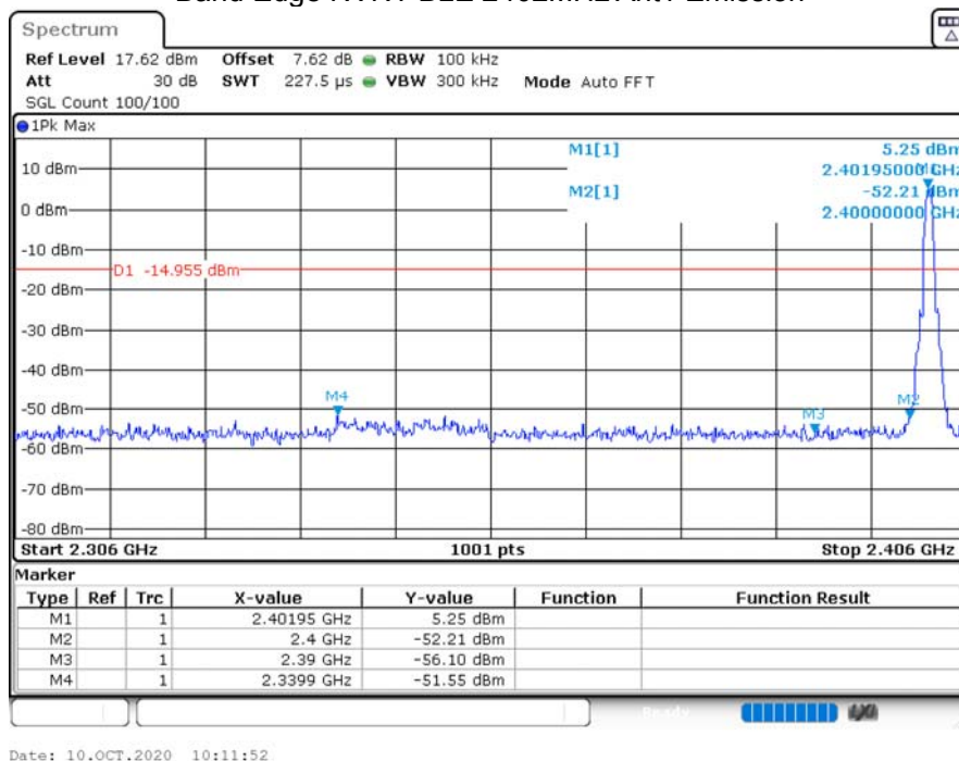
Band Edge NVNT BLE 2402MHz Ant1 Emission
