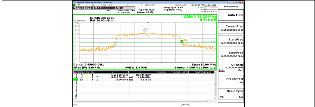
11N40SISO Ant1 5550
