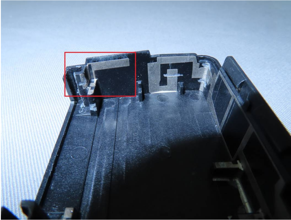
Antenna
