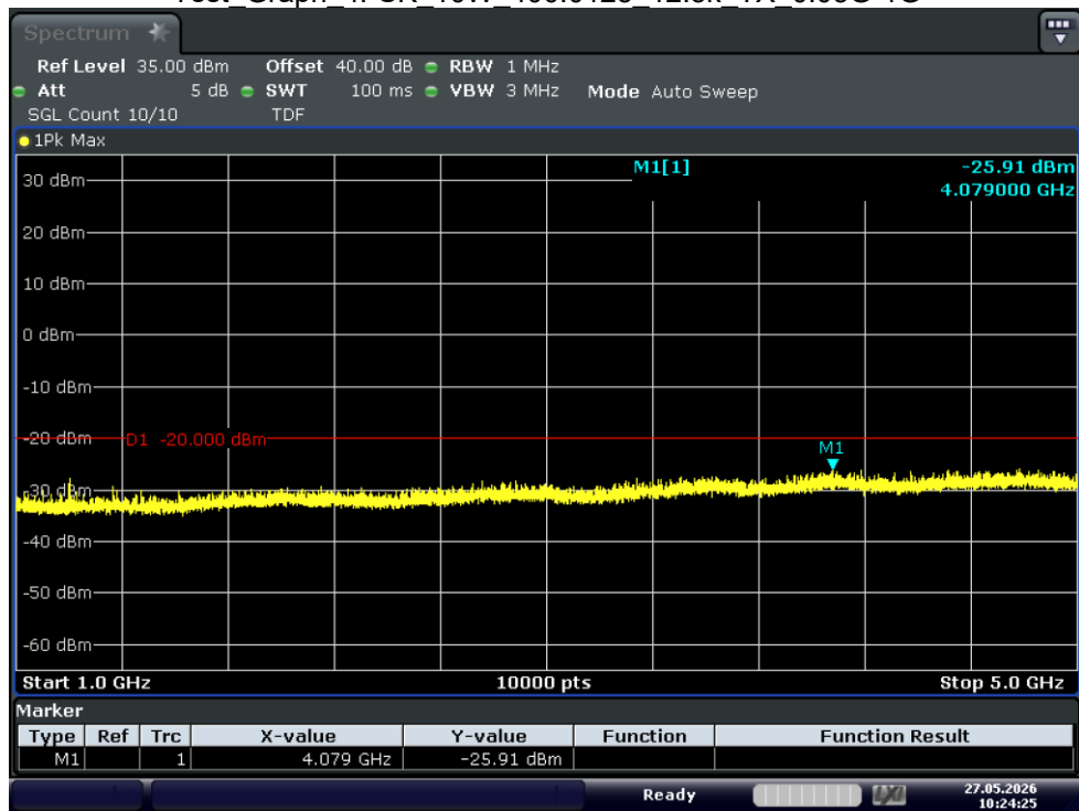
Test_Graph_4FSK_10W_400.0125_12.5k_TX_1G-5G
