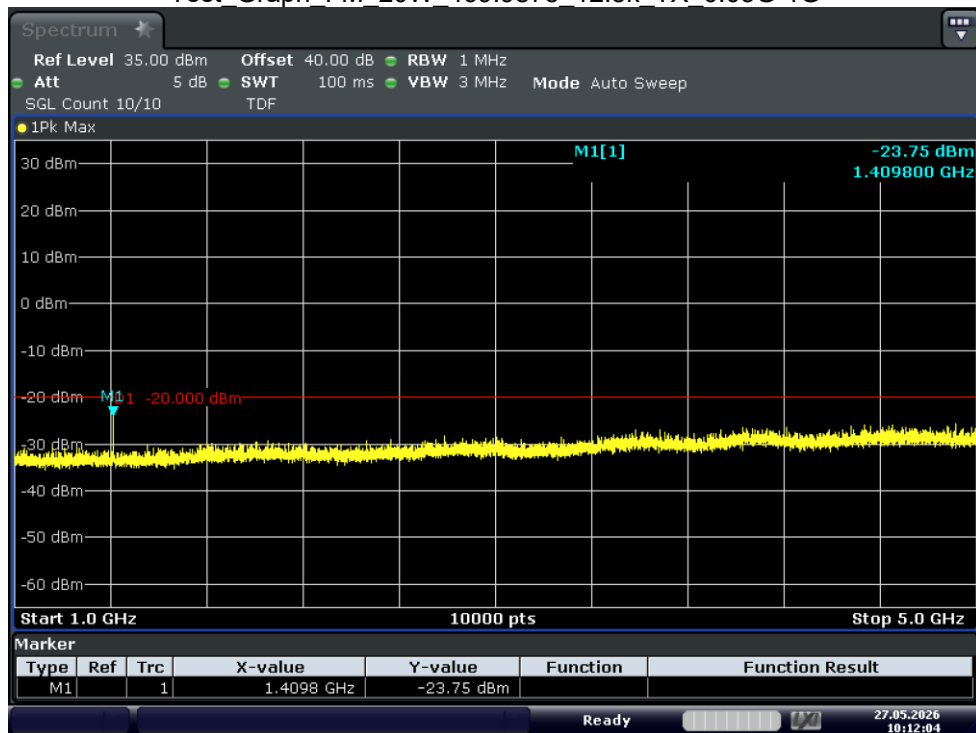
Test_Graph_FM_20W_469.9875_12.5k_TX_1G-5G
