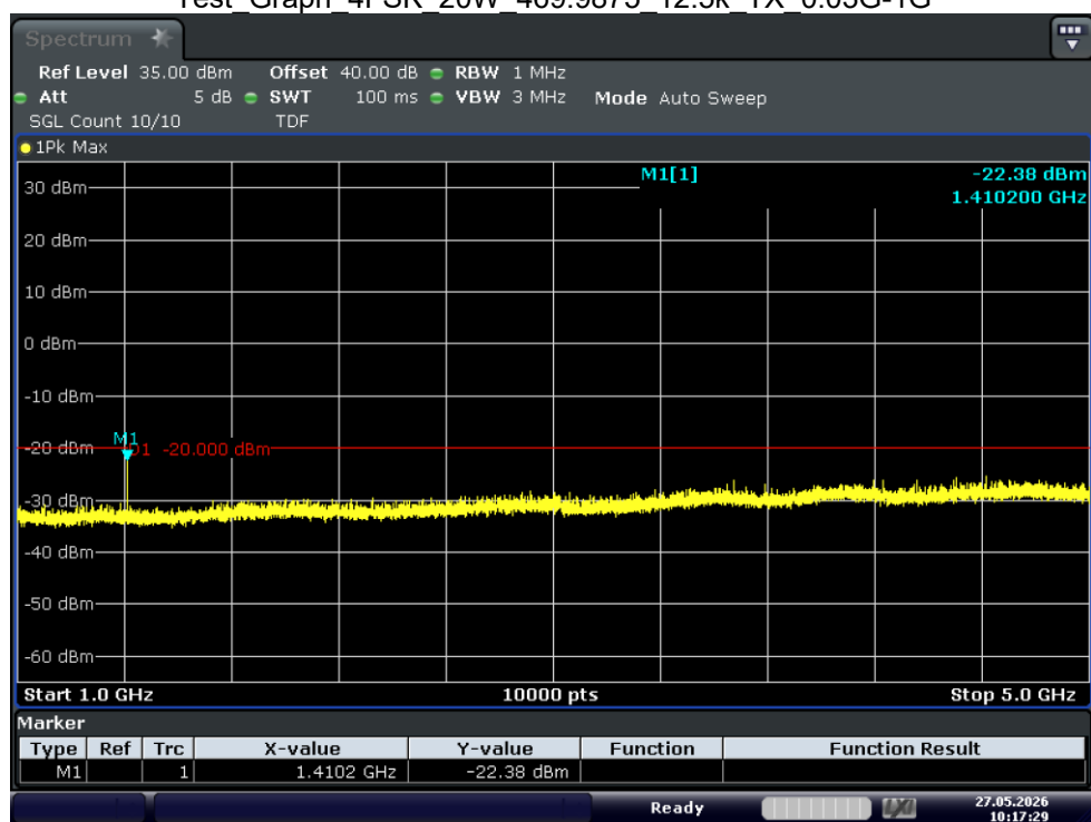
Test_Graph_4FSK_20W_469.9875_12.5k_TX_1G-5G
