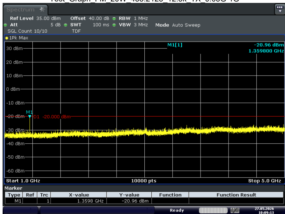
Test_Graph_FM_20W_453.2125_12.5k_TX_1G-5G
