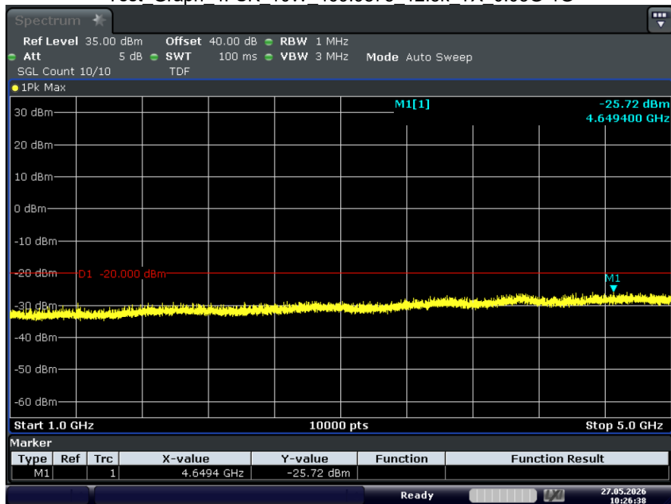
Test_Graph_4FSK_10W_469.9875_12.5k_TX_1G-5G
