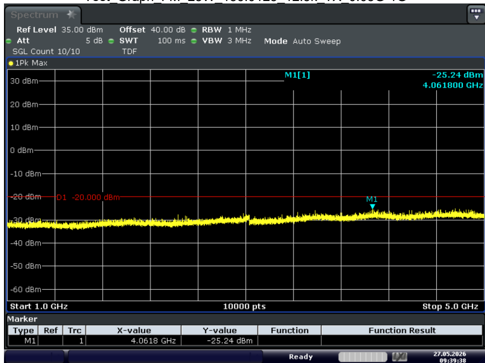
Test_Graph_FM_25W_136.0125_12.5k_TX_1G-5G
