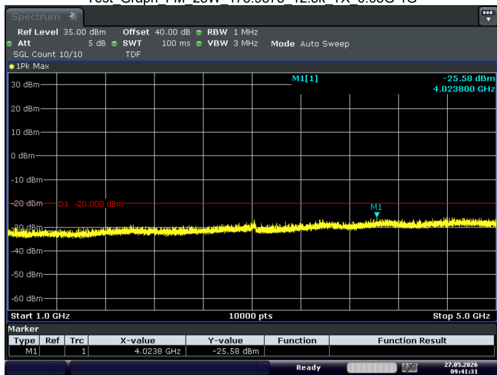
Test_Graph_FM_25W_173.9875_12.5k_TX_1G-5G
