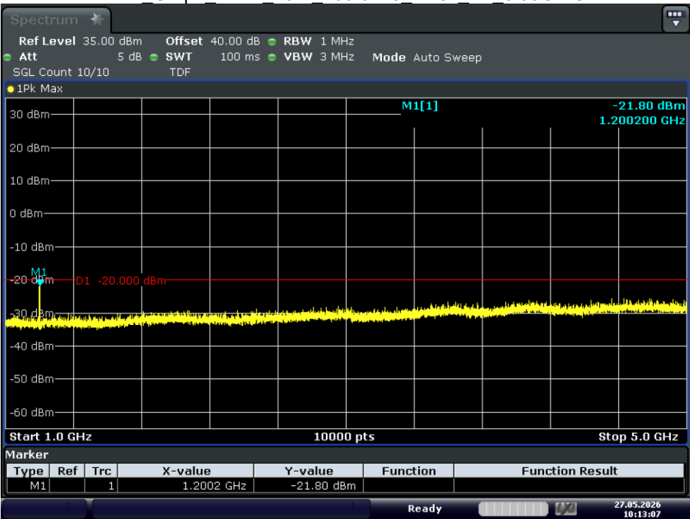
Test_Graph_4FSK_20W_400.0125_12.5k_TX_1G-5G
