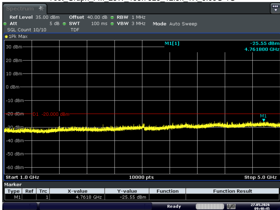
Test_Graph_FM_25W_155.7525_12.5k_TX_1G-5G
