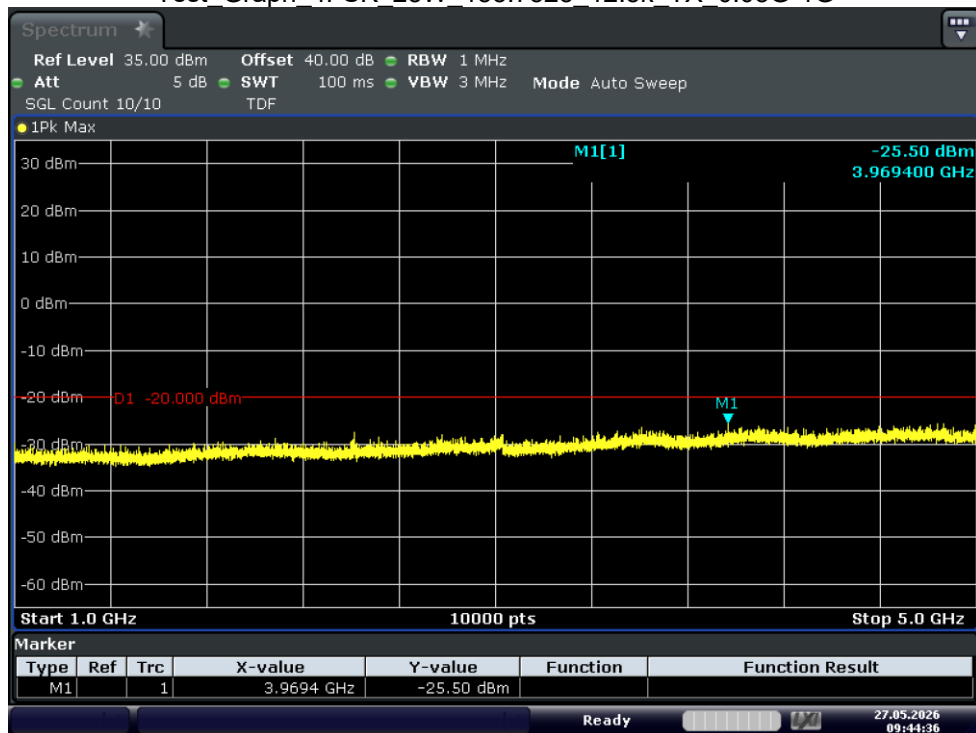
Test_Graph_4FSK_25W_155.7525_12.5k_TX_1G-5G
