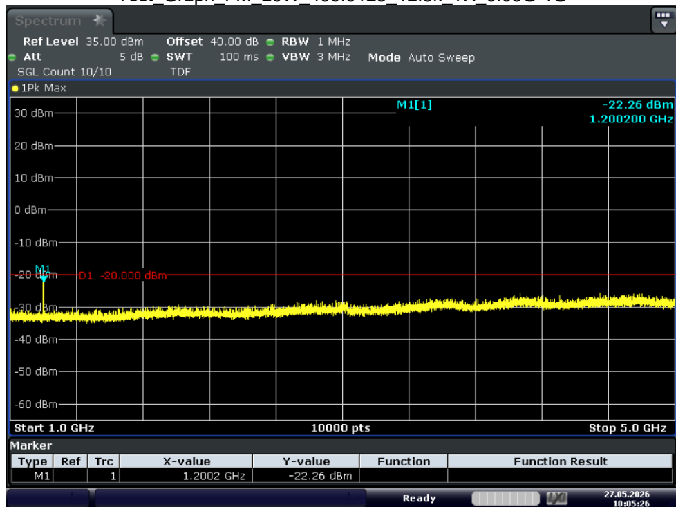
Test_Graph_FM_20W_400.0125_12.5k_TX_1G-5G
