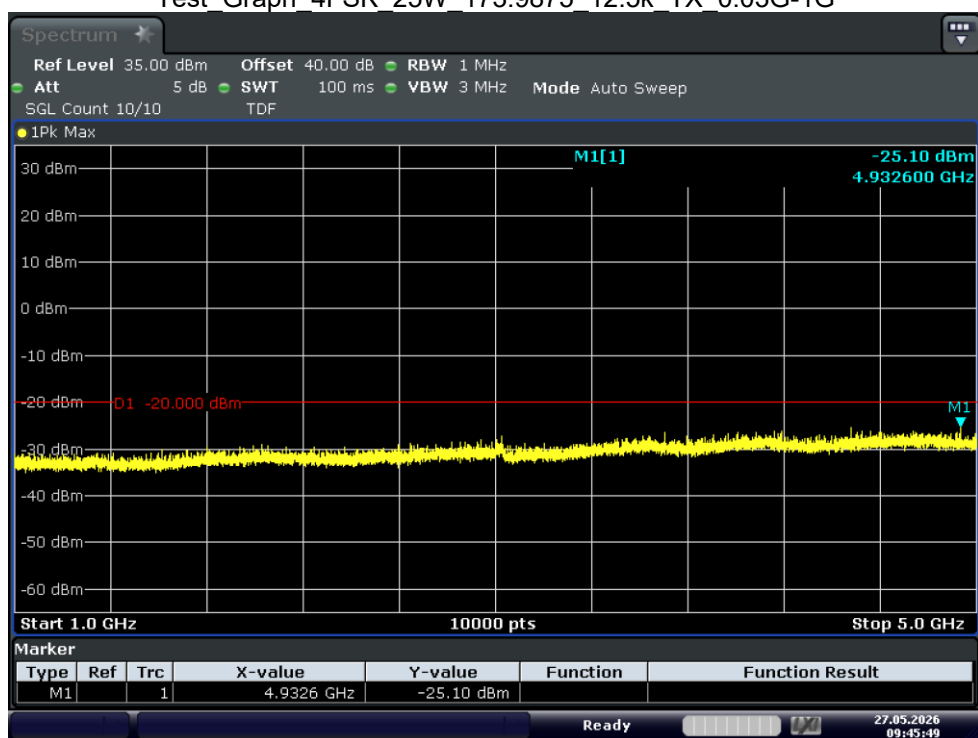
Test_Graph_4FSK_25W_173.9875_12.5k_TX_1G-5G
