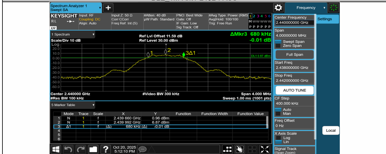
BLE 1M-Ant1-2440-PASS
