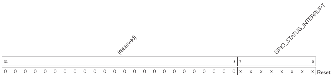
Register 4.19: GPIO_STATUS1_REG (0x0050)
