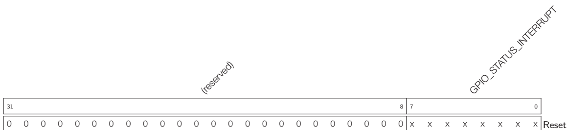
Register 4.21: GPIO_STATUS1_W1TC_REG (0x0058)
