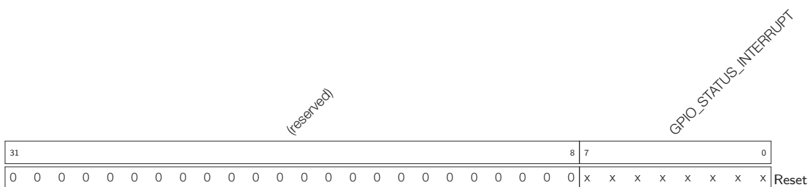
Register 4.20: GPIO_STATUS1_W1TS_REG (0x0054)
