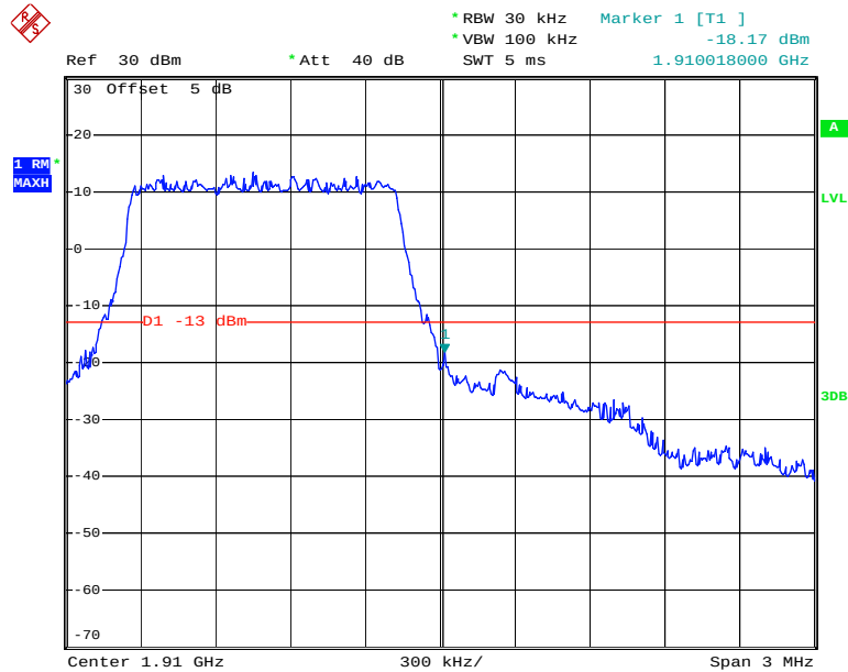
QPSK_1.4MHz_ 6 RB_ Right
