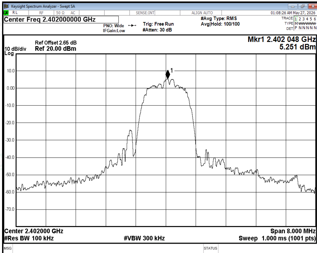
Band Edge NVNT 2-DH5 2402MHz Ant No-Hopping Ref
