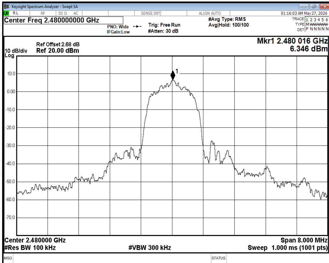
Band Edge NVNT 3-DH5 2480MHz Ant No-Hopping Ref
