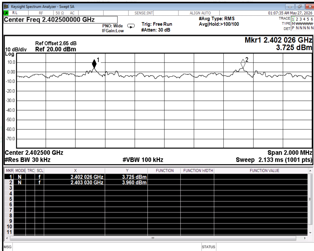
CFS NVNT 2-DH5 2402MHz Ant
