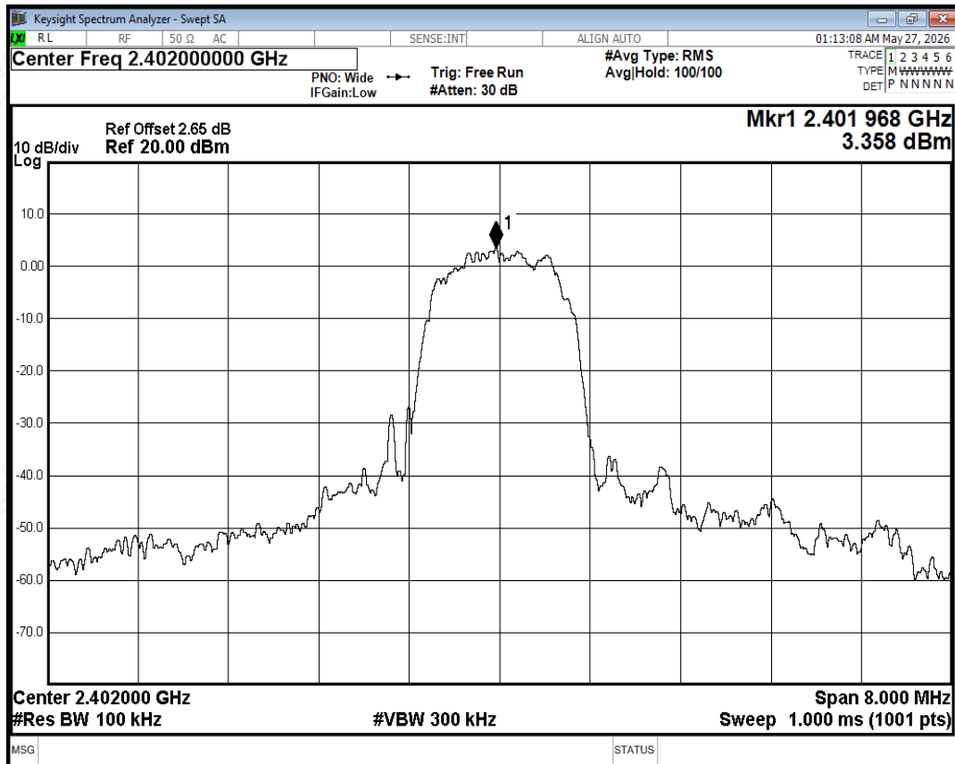
Band Edge NVNT 3-DH5 2402MHz Ant No-Hopping Ref
