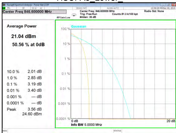
HSPA5_Higher_
