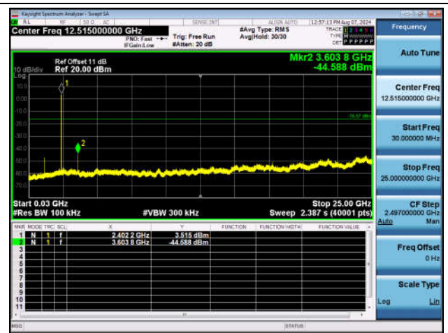
BLE_2M-Ant1-2402-30~25000-PASS
