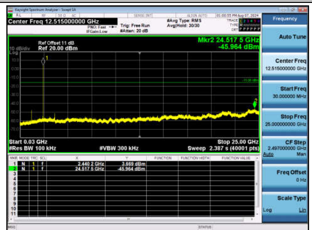
BLE_2M-Ant1-2440-30~25000-PASS
