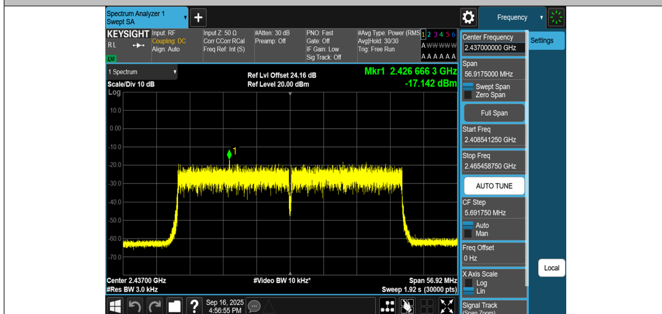
11AX40MIMO-Ant1-2437-PASS
