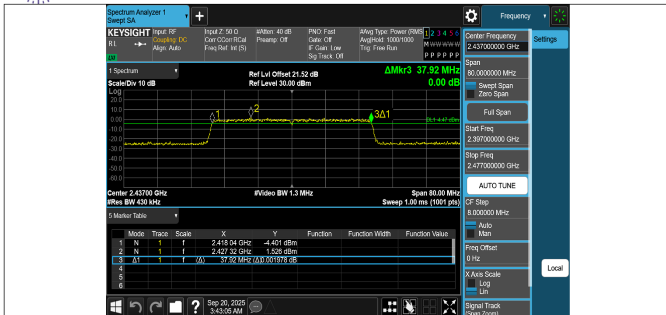
11AX40MIMO-Ant1-2437-PASS
