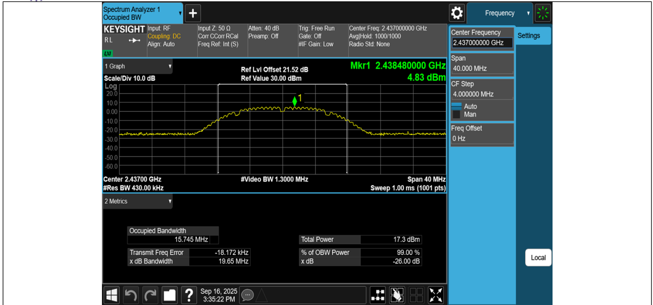
11B-Ant1-2437
