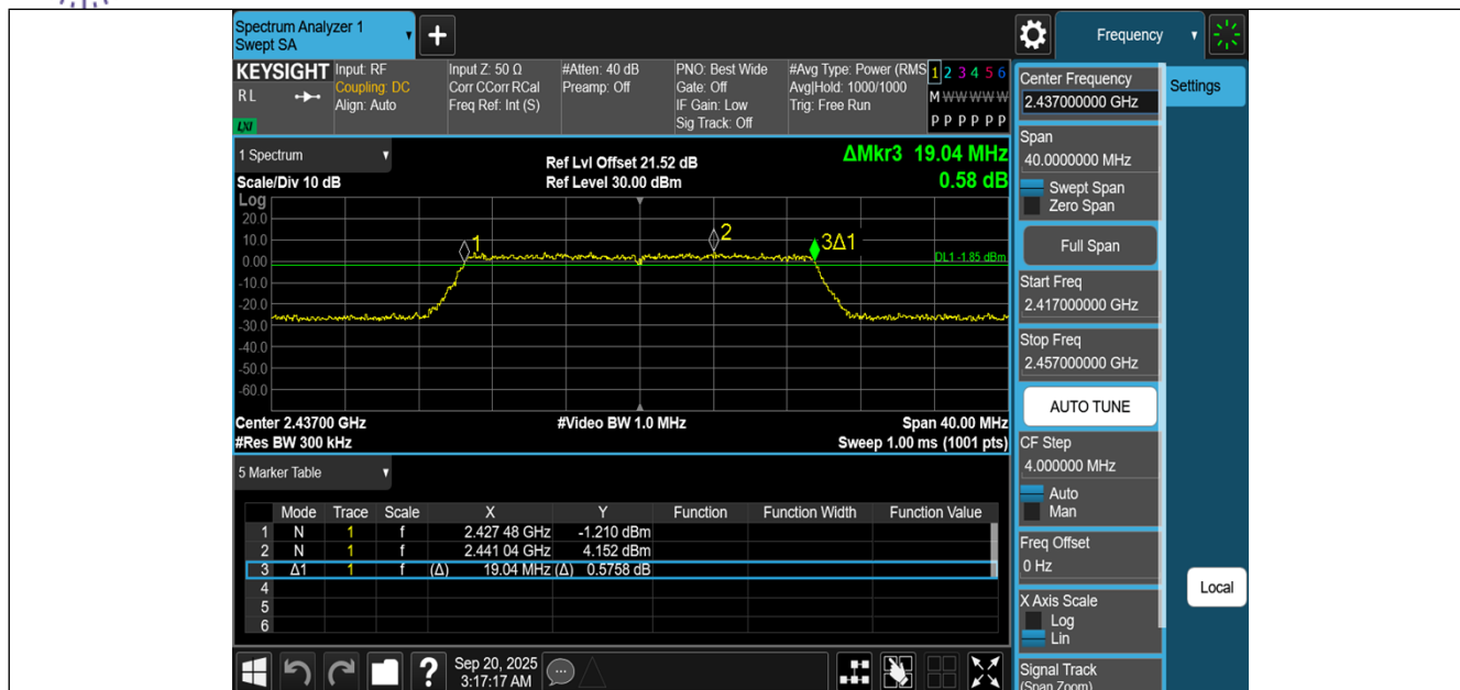
11AX20MIMO-Ant1-2437-PASS
