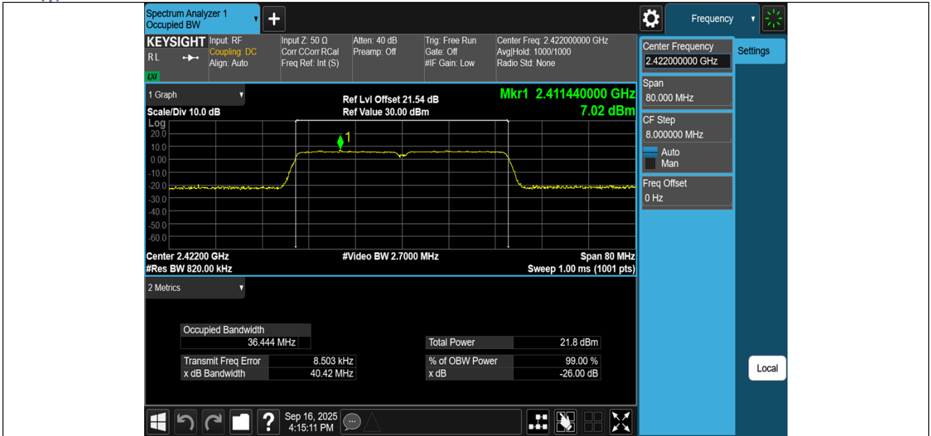
11N40MIMO-Ant1-2422
