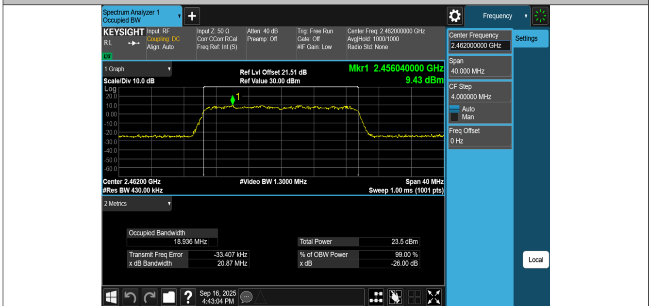
11AX20MIMO-Ant2-2462
