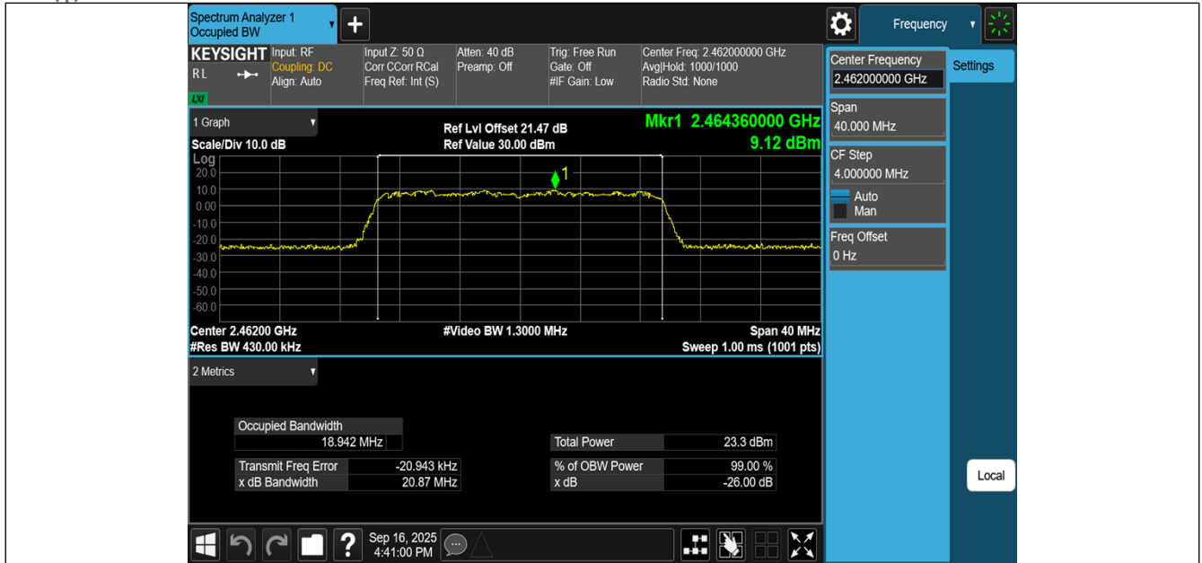
11AX20MIMO-Ant1-2462
