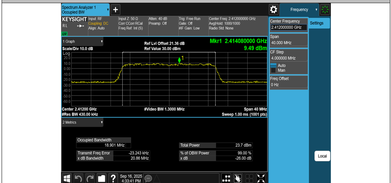
11AX20MIMO-Ant2-2412
