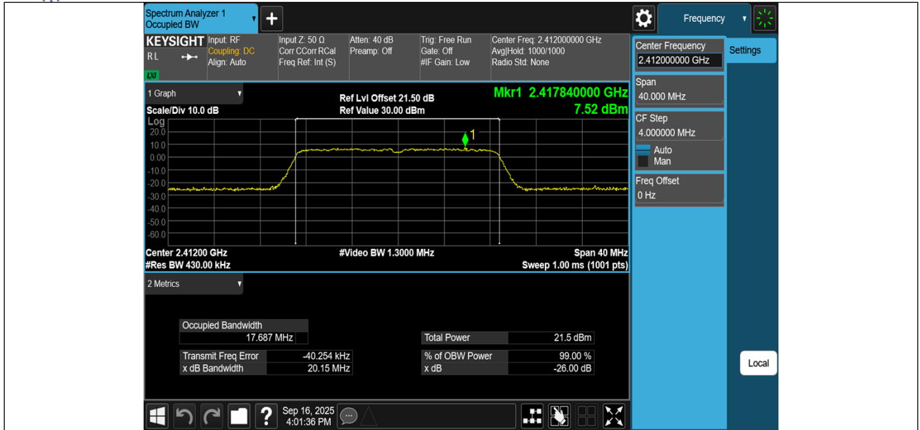
11N20MIMO-Ant1-2412
