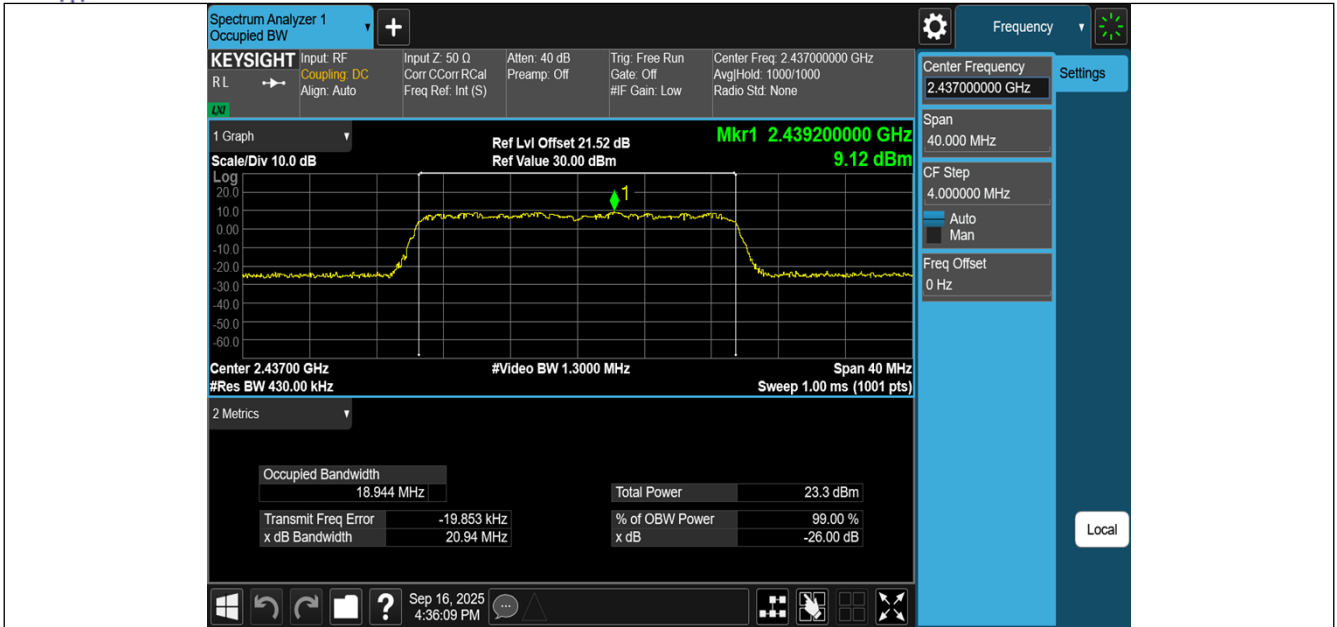
11AX20MIMO-Ant1-2437
