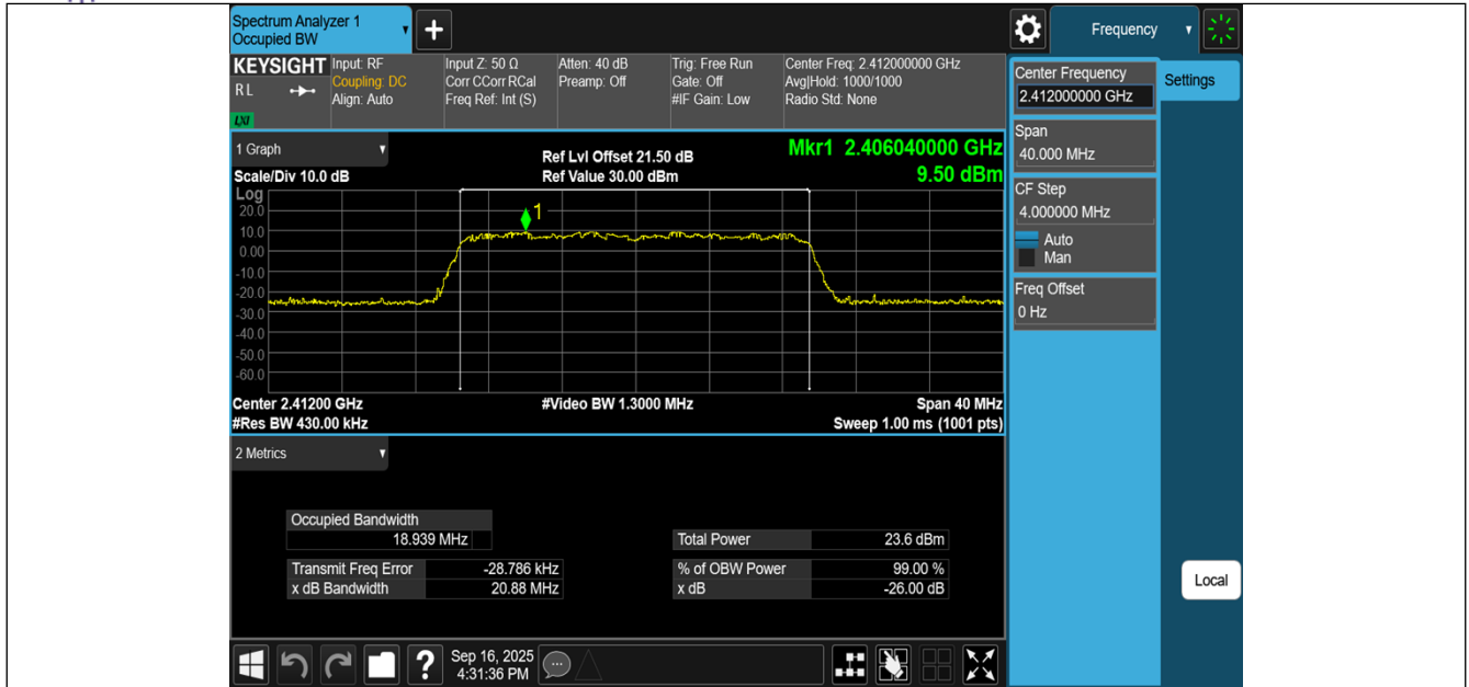
11AX20MIMO-Ant1-2412
