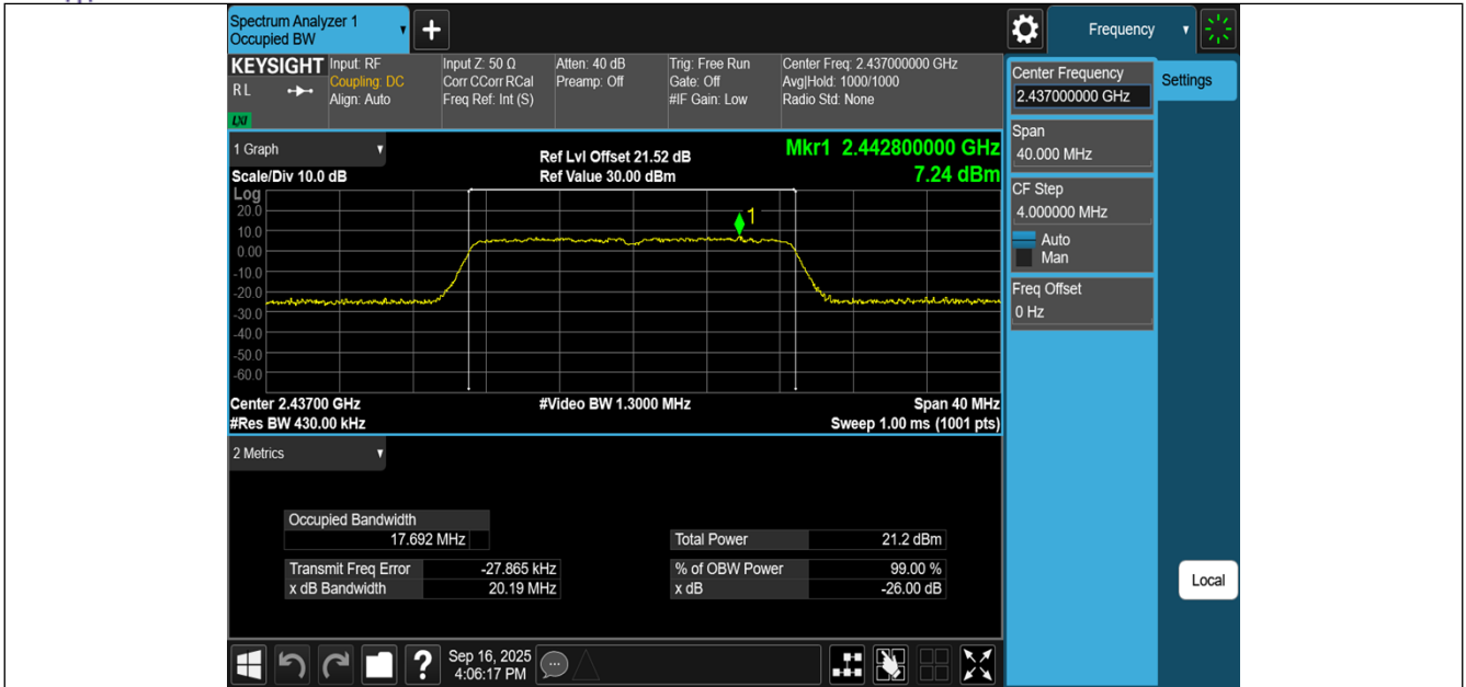
11N20MIMO-Ant1-2437
