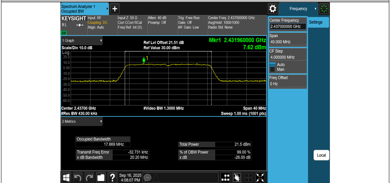
11N20MIMO-Ant2-2437
