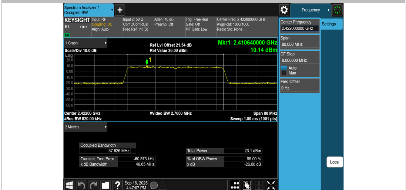
11AX40MIMO-Ant1-2422
