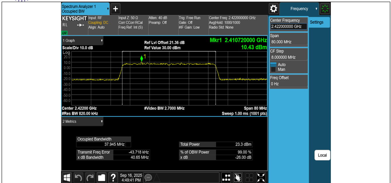
11AX40MIMO-Ant2-2422
