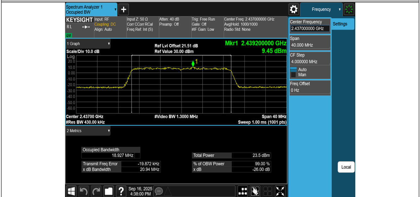
11AX20MIMO-Ant2-2437
