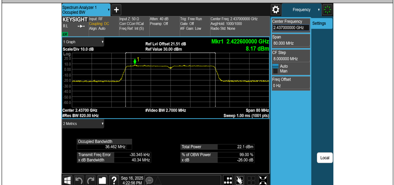
11N40MIMO-Ant2-2437
