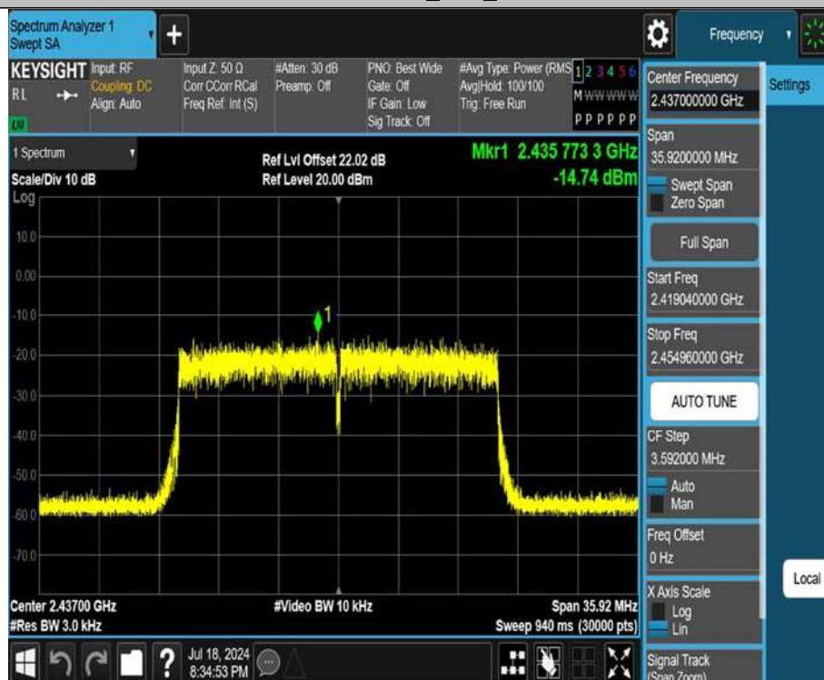
11AX20SISO_Ant1_2437
