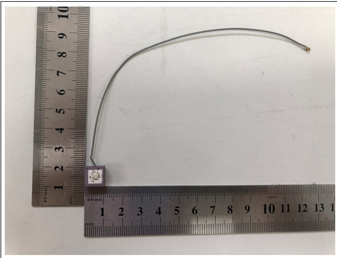
<GNSS Antenna>
