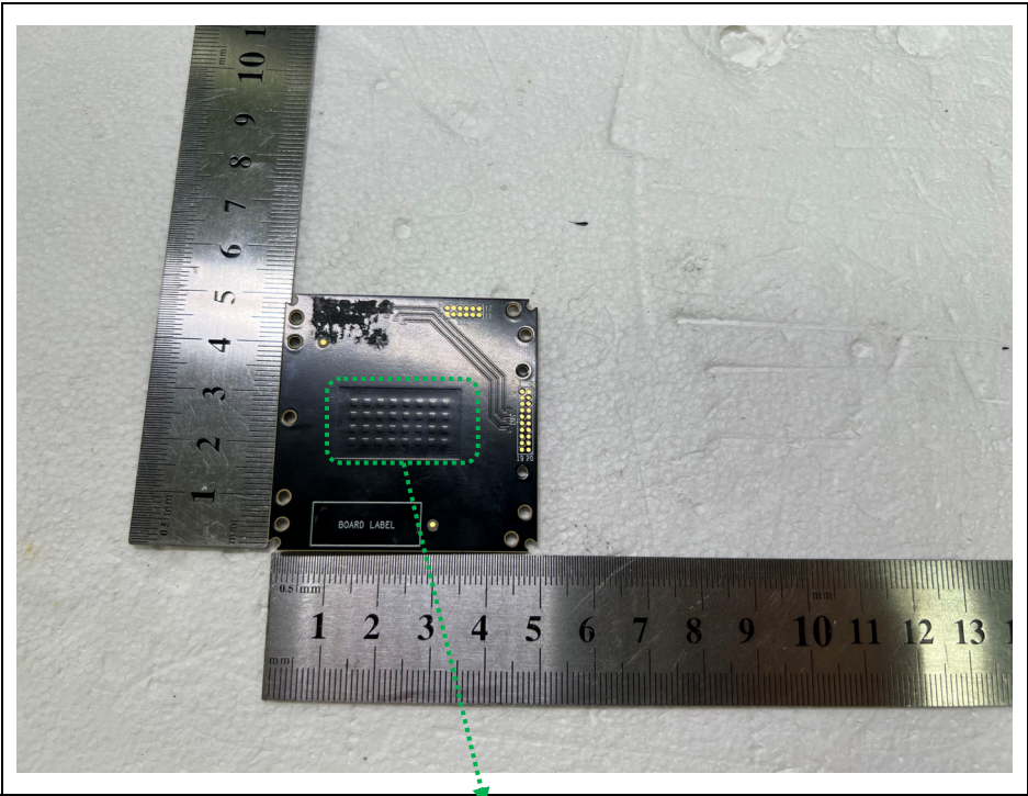
Antenna
