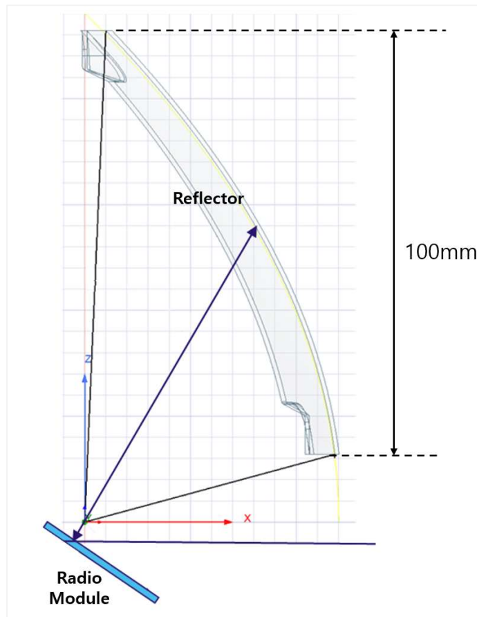
Figure 1: Reflector Antenna Parameter
