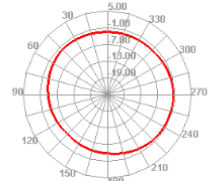
2450.000MHz H
