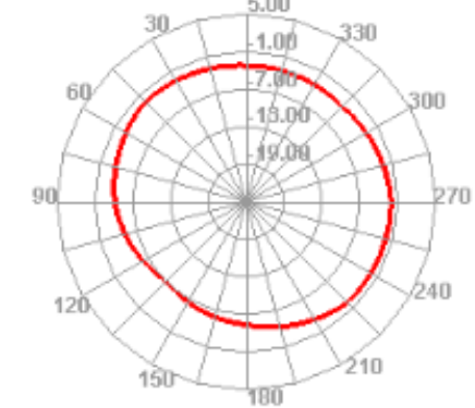
2500.000MHz H
