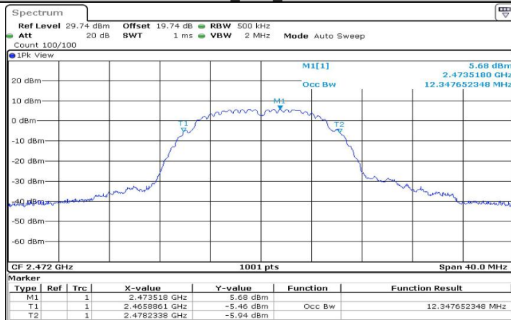
11B_Ant1_2472
