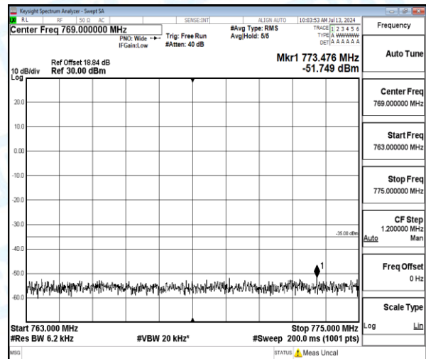
Band13-5MHz-QPSK-23230-1-0-Low-763-775-773.48--51.75-16.75--35-PASS
