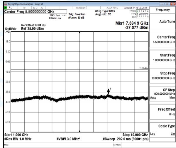
Band13-5MHz-QPSK-23205-1-0-Low-1000-10000-7384.9--37.08-24.08--13-PASS
