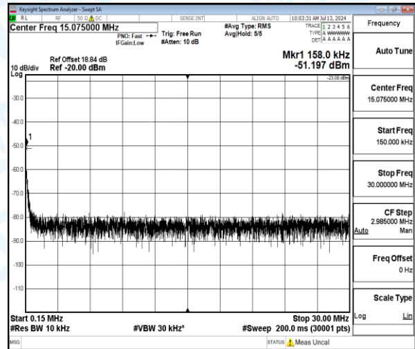
Band13-5MHz-QPSK-23230-1-0-Low-0.15-30-0.16--51.2-28.2--23-PASS
