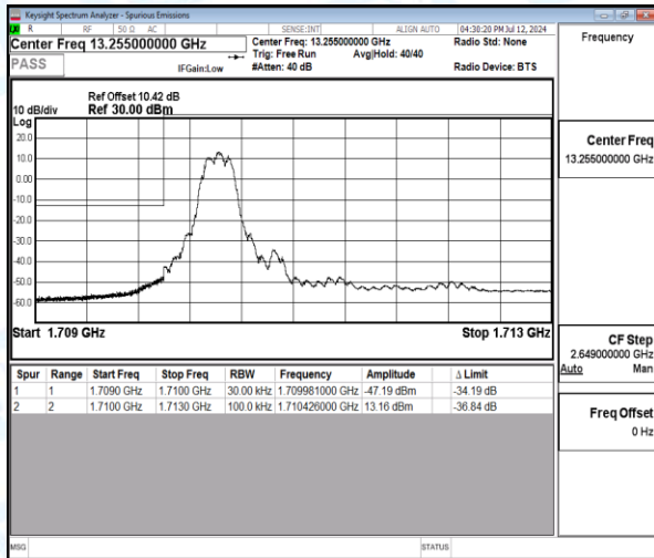
Band4-3MHz-16QAM-19965-1-0-Low-1709.98--47.19-34.19-PASS
