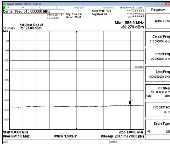
Band4-1.4MHz-QPSK-19957-1-0-Low-30-1000-899.02--50.28-37.28--13-PASS
