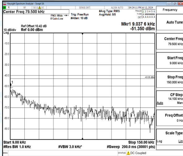
Band4-3MHz-QPSK-19965-1-0-Low-0.009-0.15-0.01--51.35-8.35--43-PASS
