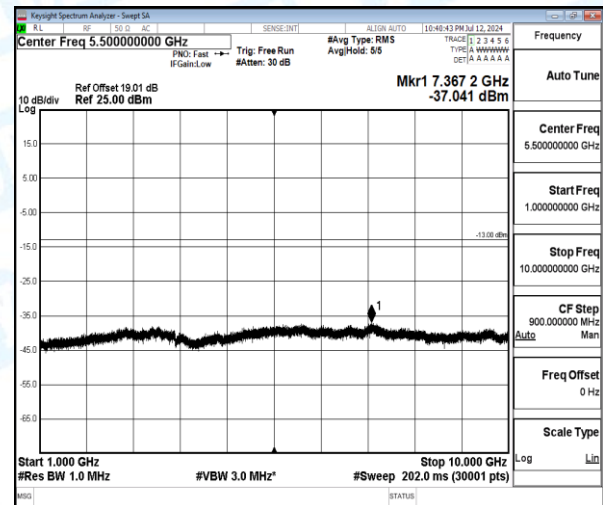
Band5-3MHz-QPSK-20415-1-0-Low-1000-10000-7367.2--37.04-24.04--13-PASS
