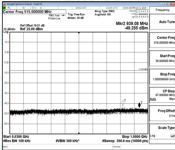
Band5-3MHz-16QAM-20415-1-0-Low-30-1000-939.08--49.26-36.26--13-PASS
