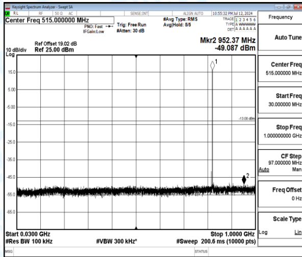
Band5-5MHz-QPSK-20425-1-0-Low-30-1000-952.37--49.09-36.09--13-PASS
