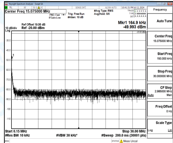
Band5-3MHz-QPSK-20525-1-0-Low-0.15-30-0.16--49.99-26.99--23-PASS
