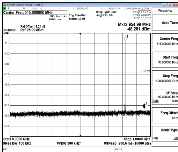
Band5-3MHz-QPSK-20415-1-0-Low-30-1000-954.99--48.28-35.28--13-PASS
