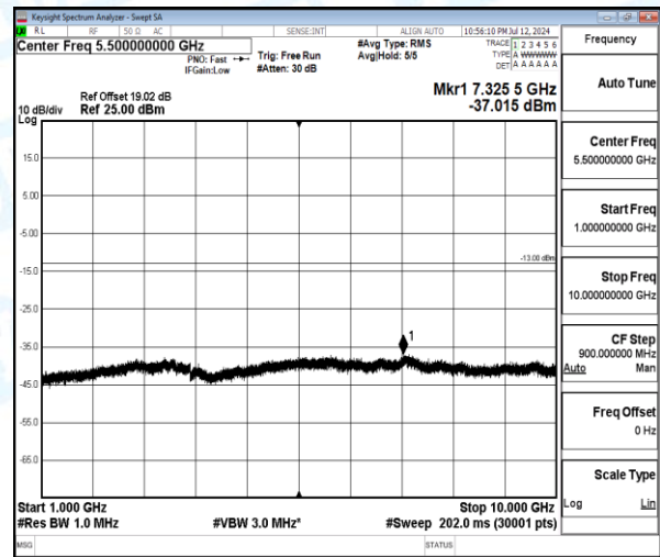
Band5-5MHz-16QAM-20425-1-0-Low-1000-10000-7325.5--37.02-24.02--13-PASS
