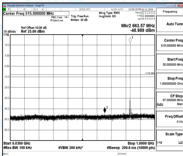
Band5-5MHz-QPSK-20525-1-0-Low-30-1000-663.57--48.99-35.99--13-PASS
