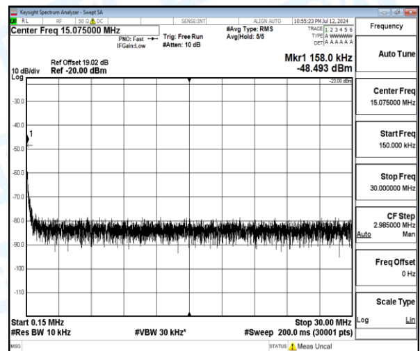
Band5-5MHz-QPSK-20425-1-0-Low-0.15-30-0.16--48.49-25.49--23-PASS
