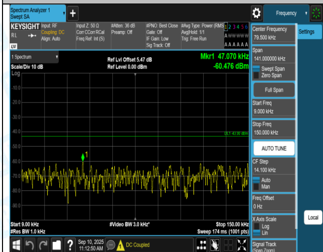
Band2-20MHz-QPSK-19100-100RB#0-30-1000-PASS
