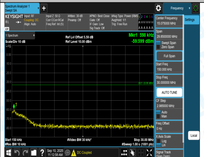
Band2-20MHz-QPSK-19100-100RB#0-1000-3000-PASS
