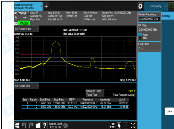
Band2-3MHz-QPSK-18615-15RB#0-PASS
