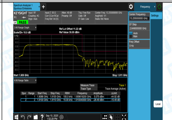
Band2-3MHz-QPSK-18615-1RB#14-PASS
