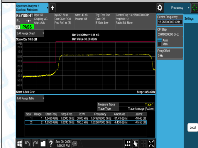
Band2-3MHz-QPSK-19185-1RB#14-PASS
