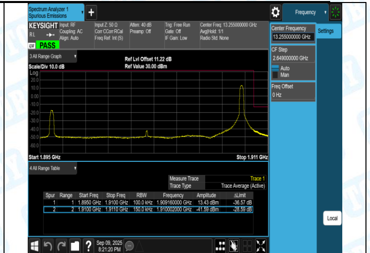
Band2-20MHz-QPSK-18700-1RB#99-PASS
