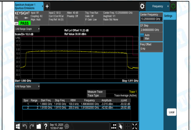
Band2-20MHz-16QAM-18700-1RB#99-PASS
