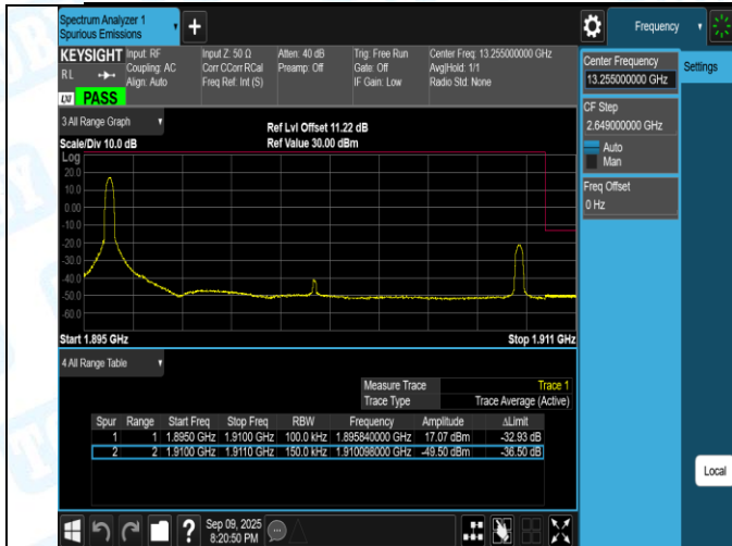
Band2-20MHz-QPSK-18700-1RB#0-PASS
