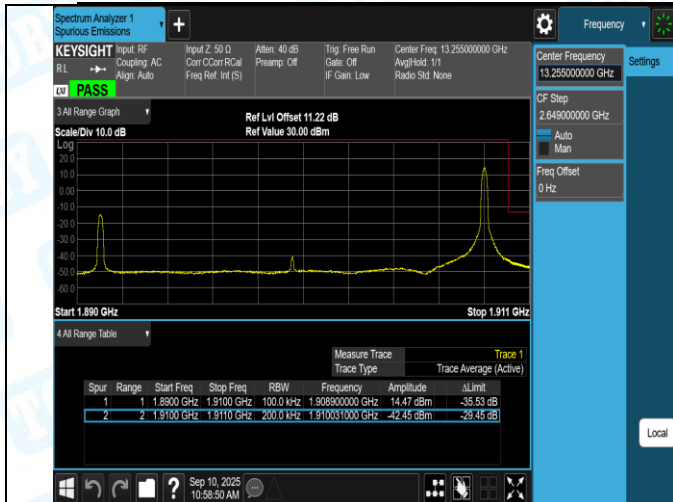
Band2-20MHz-16QAM-18700-1RB#0-PASS
