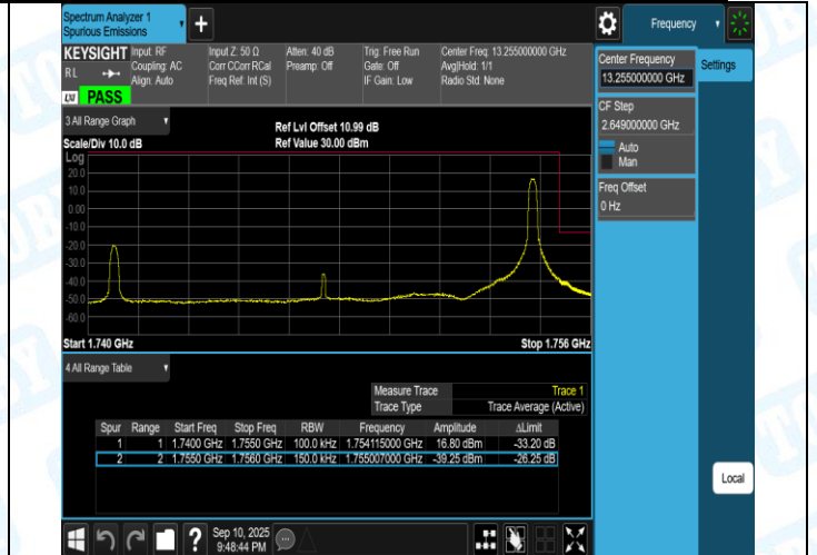
Band4-20MHz-QPSK-20050-1RB#99-PASS
