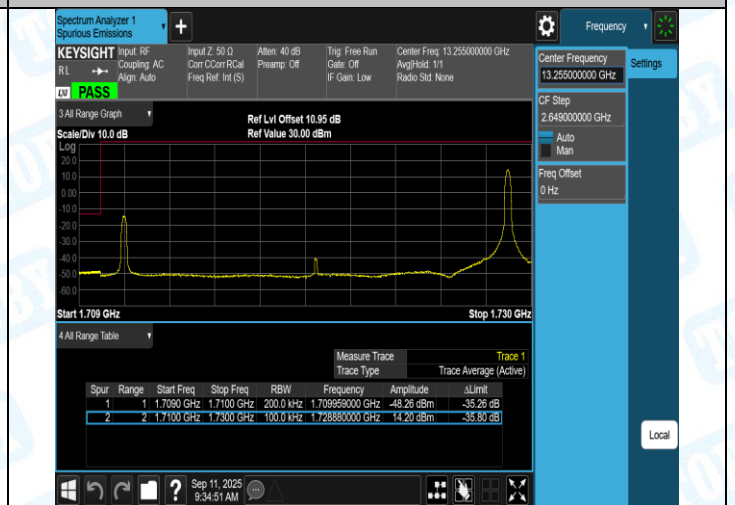
Band4-20MHz-QPSK-20050-100RB#99-PASS
