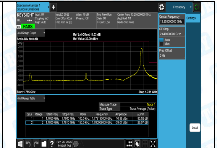
Band66-20MHz-QPSK-132072-1RB#99-PASS
