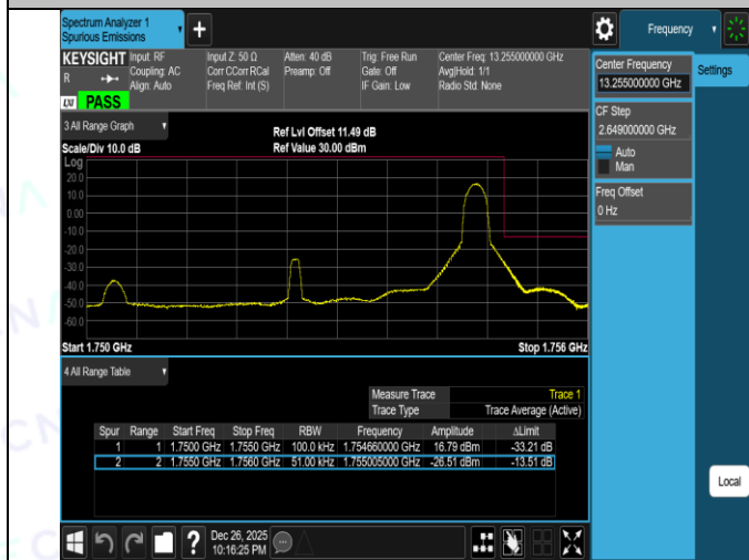
Band4-10MHz-QPSK-20000-1RB#0-PASS
