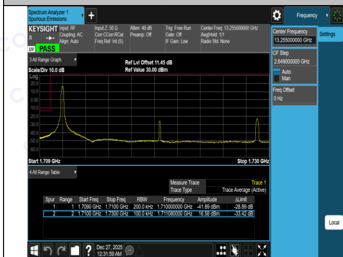
Band4-20MHz-QPSK-20050-100RB#0-PASS
