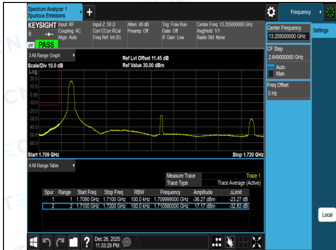
Band4-10MHz-QPSK-20000-50RB#0-PASS
