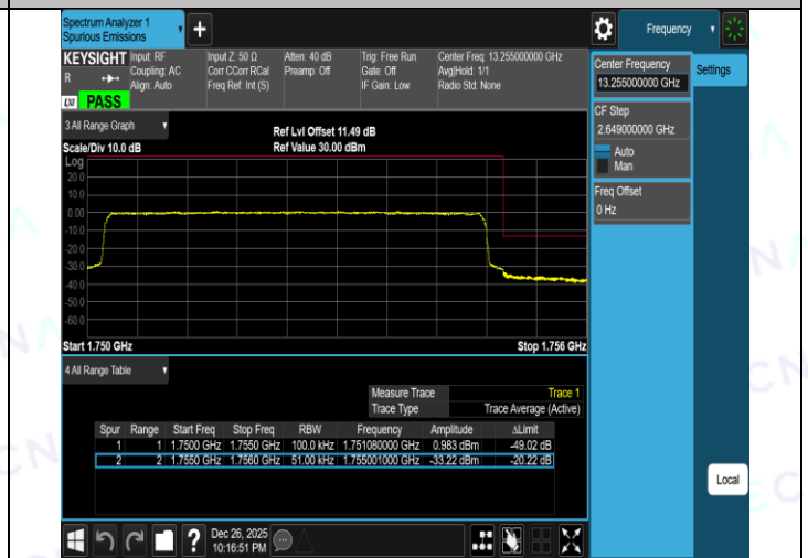
Band4-10MHz-QPSK-20000-1RB#49-PASS
