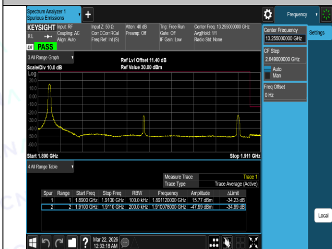
Band2-20MHz-16QAM-19100-1RB#0-PASS
