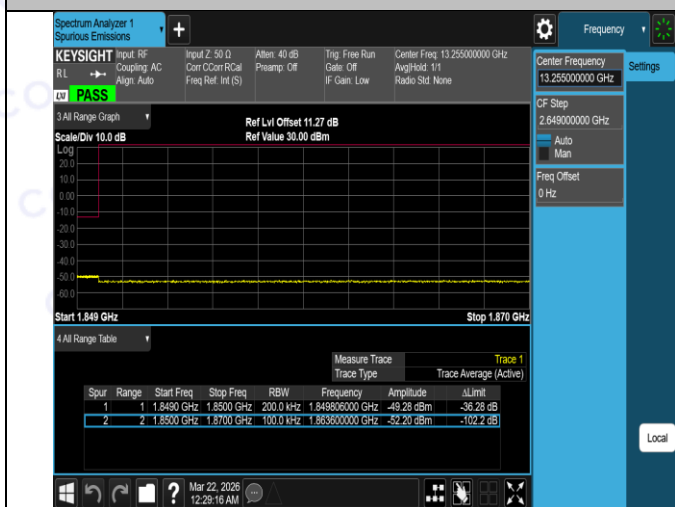
Band2-20MHz-QPSK-18700-100RB#0-PASS
