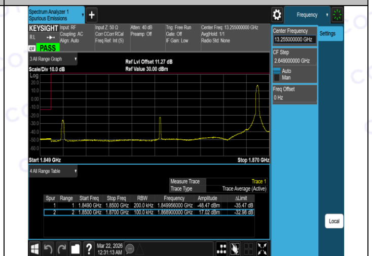
Band2-20MHz-QPSK-18700-100RB#99-PASS
