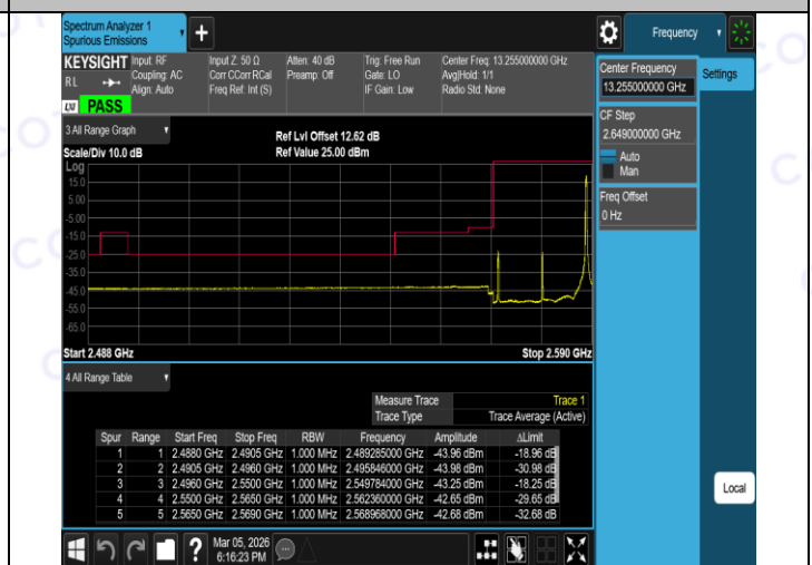
Band38-20MHz-QPSK-38150-1RB#0-PASS
