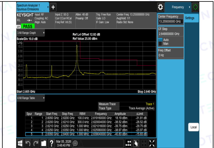
Band38-20MHz-QPSK-37850-1RB#99-PASS
