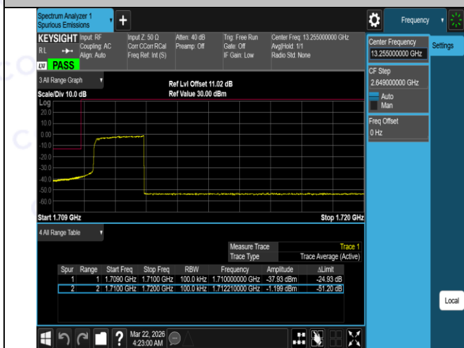
Band4-10MHz-QPSK-20350-1RB#49-PASS
