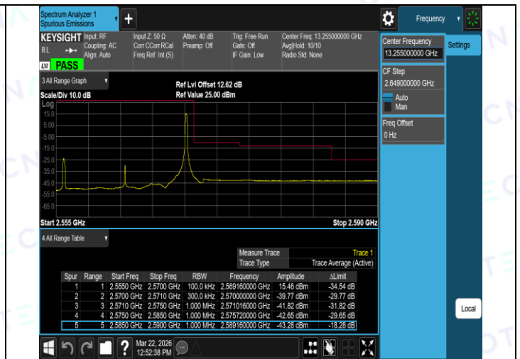
Band7-20MHz-QPSK-20850-1RB#99-PASS
