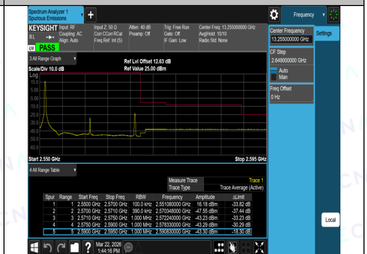
Band7-20MHz-QPSK-21350-1RB#99-PASS
