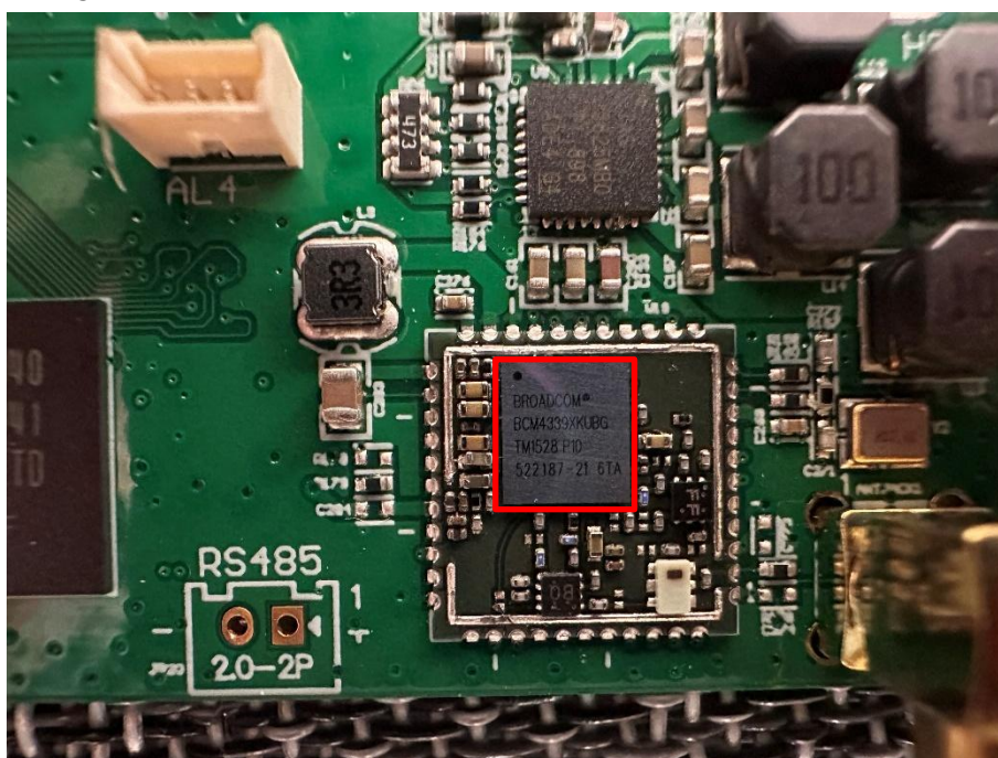
RF IC
